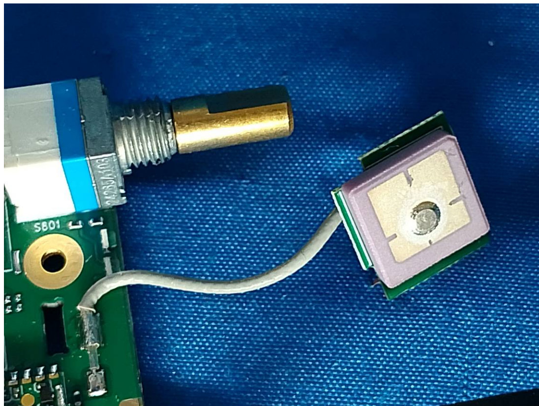
GPS Antenna
