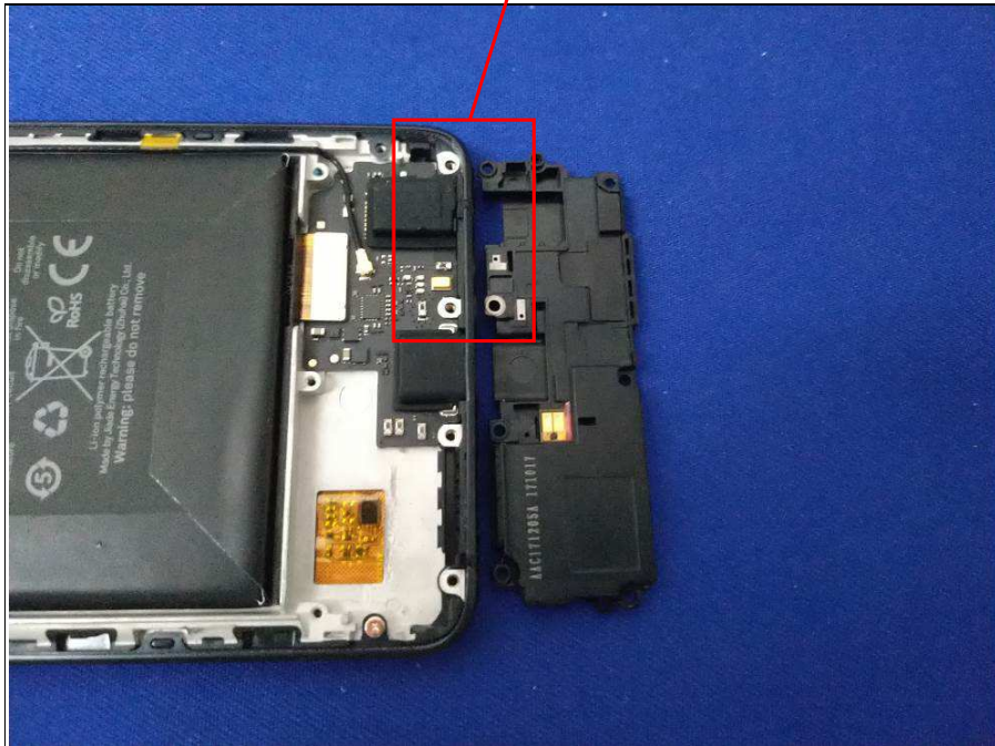
BT/WIFI/GPS Antenna
