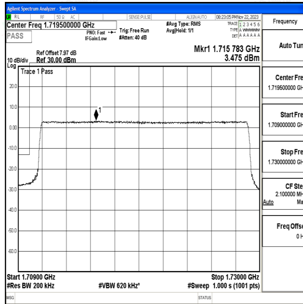
Band66_20MHz_QPSK_132072_100RB#0
