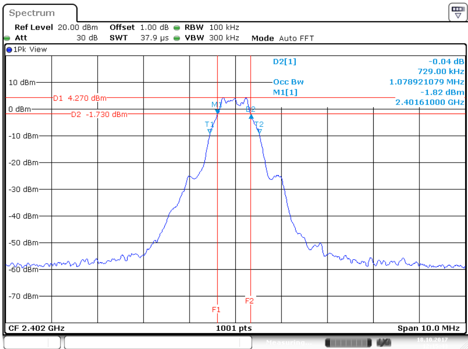
BLE Mode Low Channel
