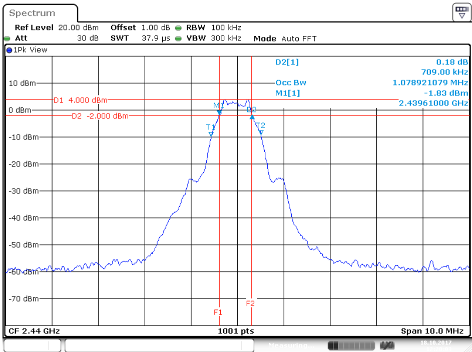
BLE Mode Middle Channel
