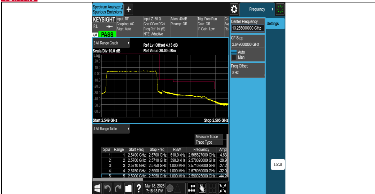
Band7-20MHz-QPSK-21350-1RB#99-PASS
