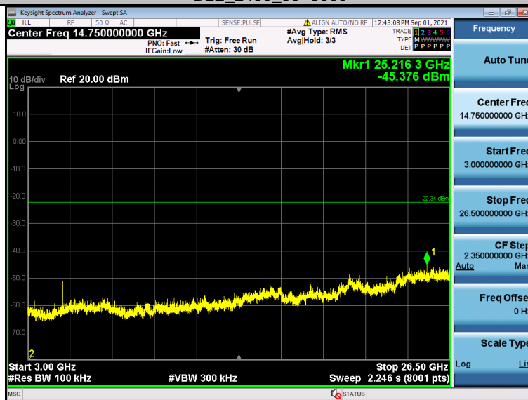
BLE_2480_3000-26500
