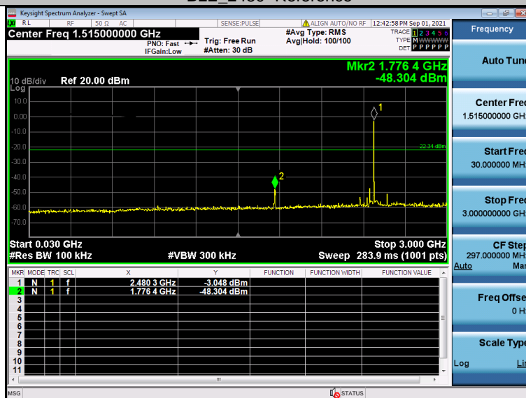
BLE_2480_30-3000
