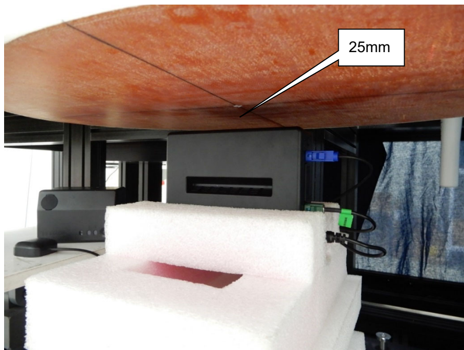
EUT Bottom_25mm
