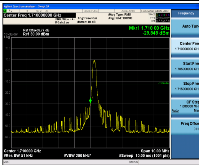
Band4-1.4MHz-16QAM-19957-1-0-Low--29.85-PASS
