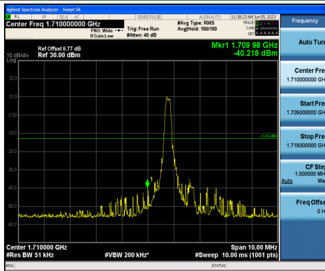
Band4-10MHz-QPSK-20000-1-0-Low--40.22-PASS
