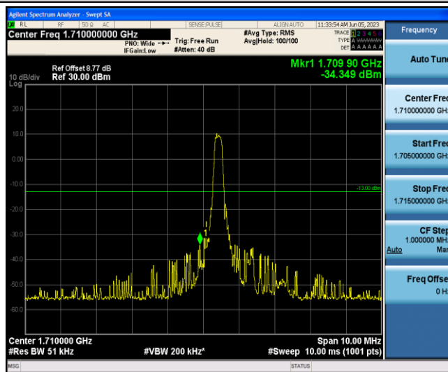
Band4-3MHz-QPSK-19965-1-0-Low--34.35-PASS
