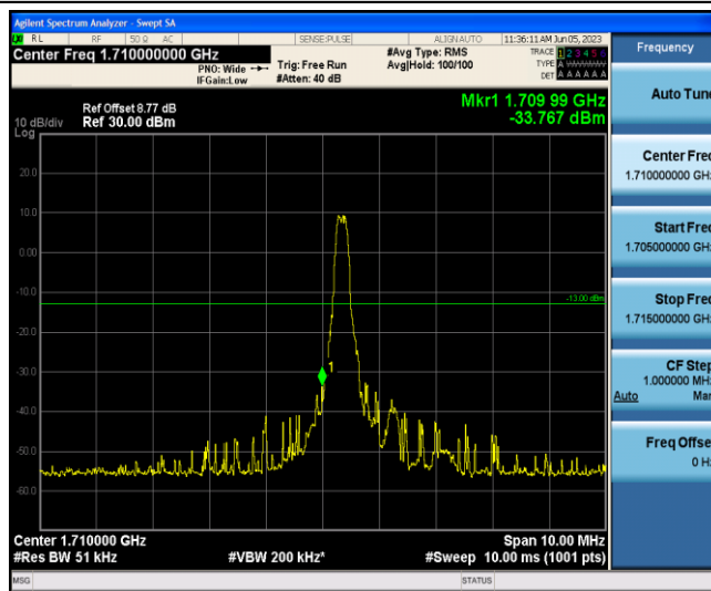
Band4-5MHz-QPSK-19975-1-0-Low--33.77-PASS
