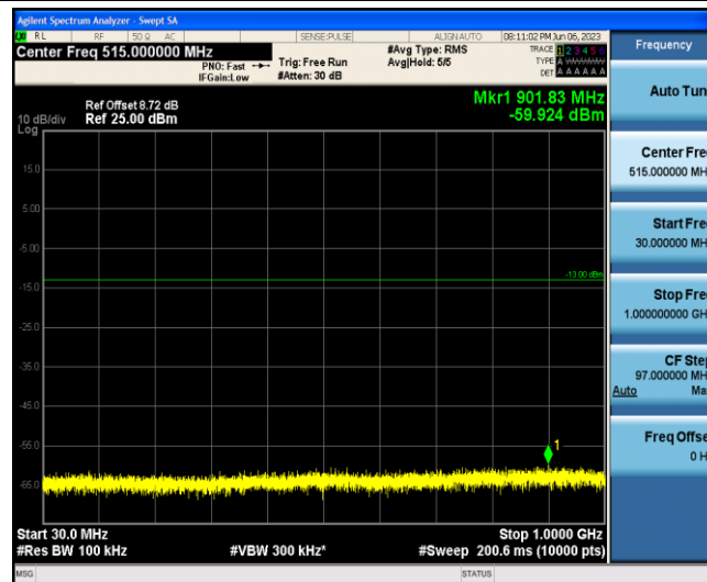
Band2-10MHz-QPSK-18650-1-0-Low-30-1000--59.92-PASS
