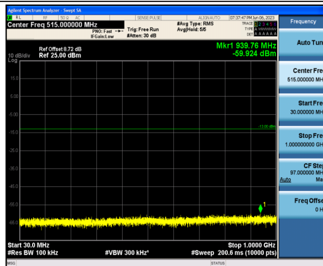
Band2-3MHz-16QAM-18900-1-0-Low-30-1000--59.92-PASS
