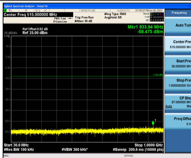
Band2-5MHz-QPSK-19175-1-0-Low-30-1000--59.48-PASS
