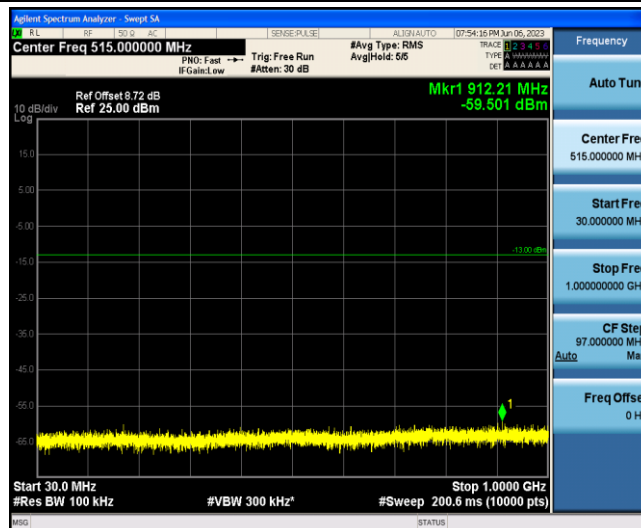
Band2-5MHz-QPSK-18900-1-0-Low-30-1000--59.5-PASS
