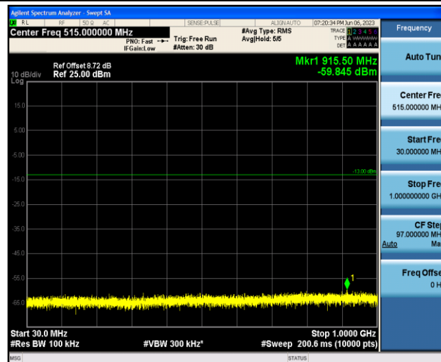
Band2-1.4MHz-QPSK-18900-1-0-Low-30-1000--59.85-PASS
