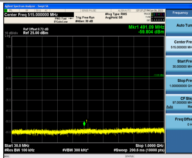
Band2-3MHz-QPSK-18900-1-0-Low-30-1000--59.8-PASS
