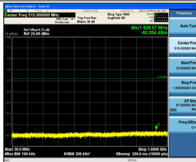
Band2-10MHz-QPSK-18900-1-0-Low-30-1000--60.05-PASS
