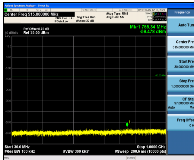
Band2-3MHz-QPSK-18615-1-0-Low-30-1000--59.48-PASS
