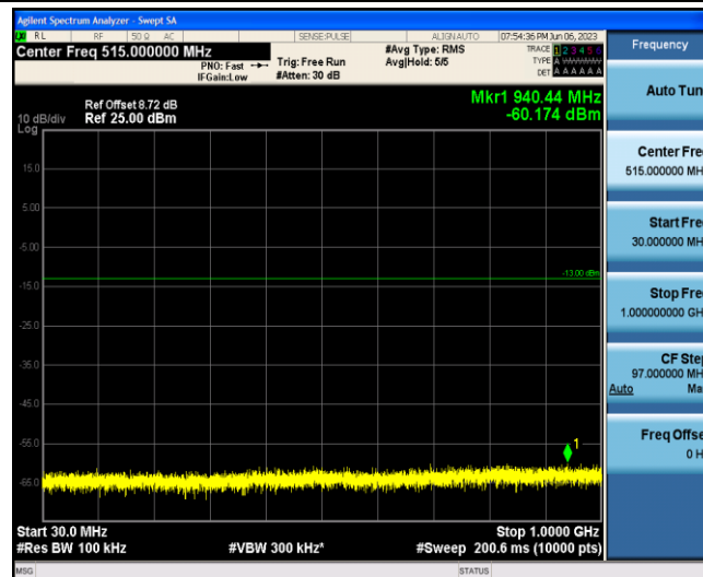
Band2-5MHz-16QAM-18900-1-0-Low-30-1000--60.17-PASS
