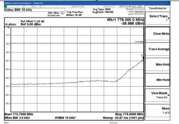
Upper 700MHz band GSM UL Left Side 10dB Above AGC
