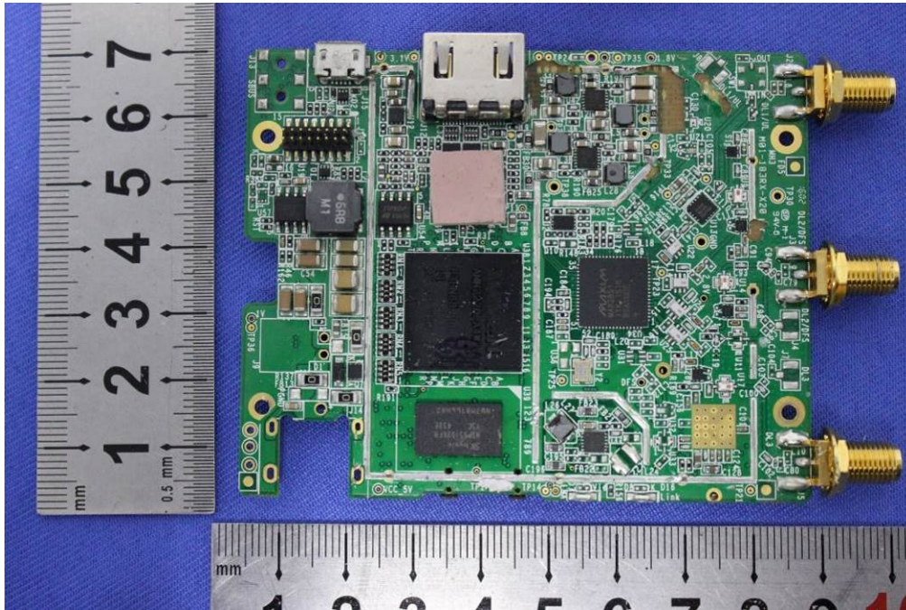
Certified Module (FCC ID: VQSAMNPTRX01)
