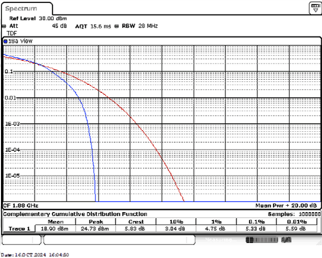
Band2-20MHz-16QAM-18900-25RB#0
