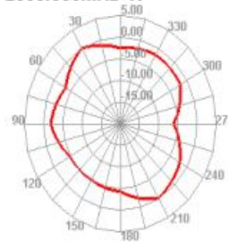
2500.000MHz H
