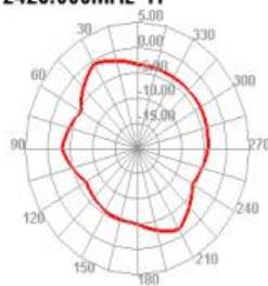
2425.000MHz H
