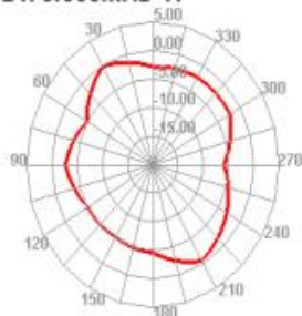
2475.000MHz E2
