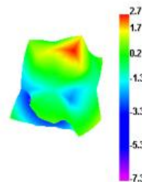
2450.000MHz E1
