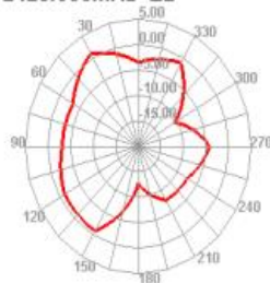
2425.000MHz E2
