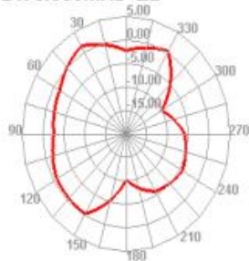
2475.000MHz E2
