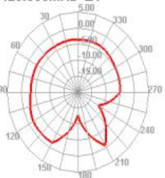
2425.000MHz E1
