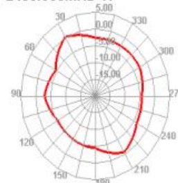
2450.000MHz E2
