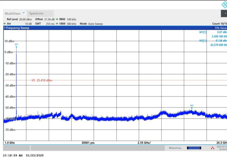
11B_Ant1_2462_0~Reference
