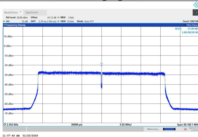
11AX40SISO_Ant1_2452
