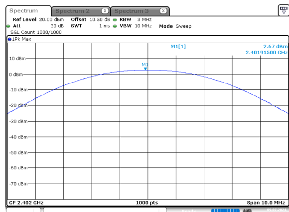
BLE 1Mbps Low
