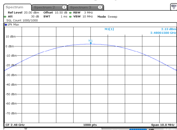
BLE 1Mbps High
