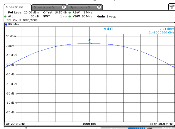
BLE 2Mbps High
