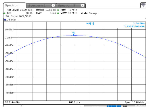
BLE 1Mbps Middle
