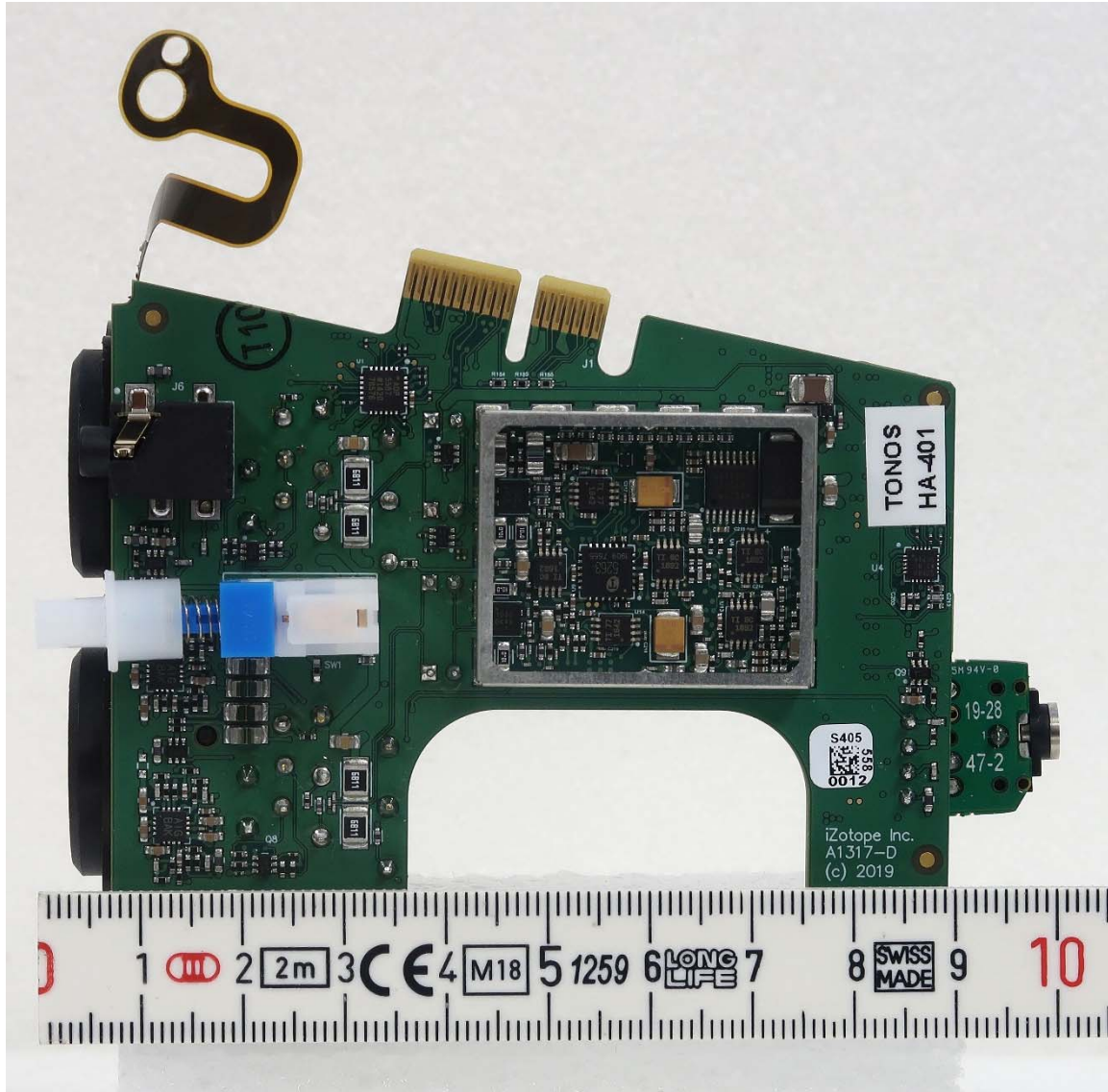
Tonos HA – 401 Audio Module side 1
