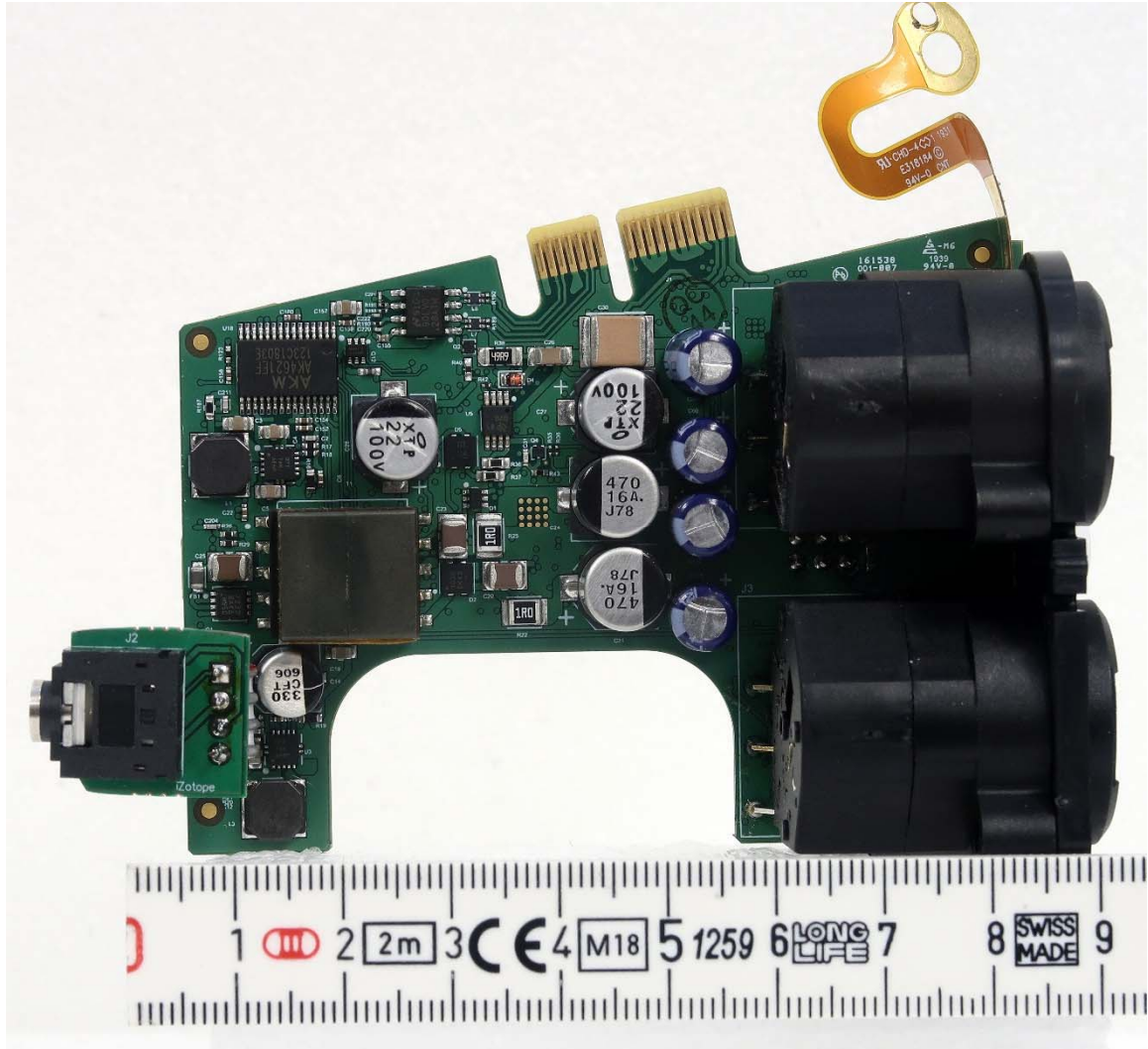
Tonos HA – 401 Audio Module side 2
