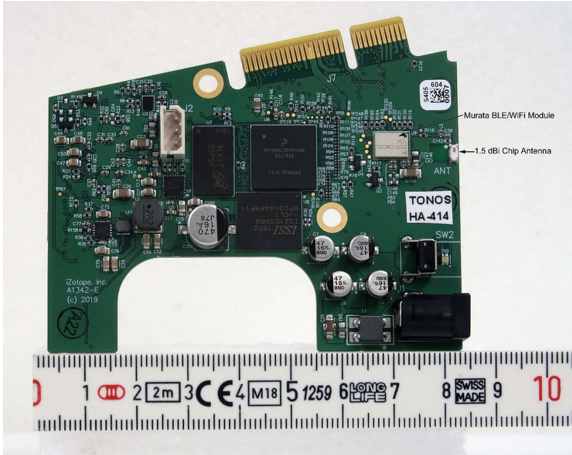
Tonos HA – 414 Module side 2
