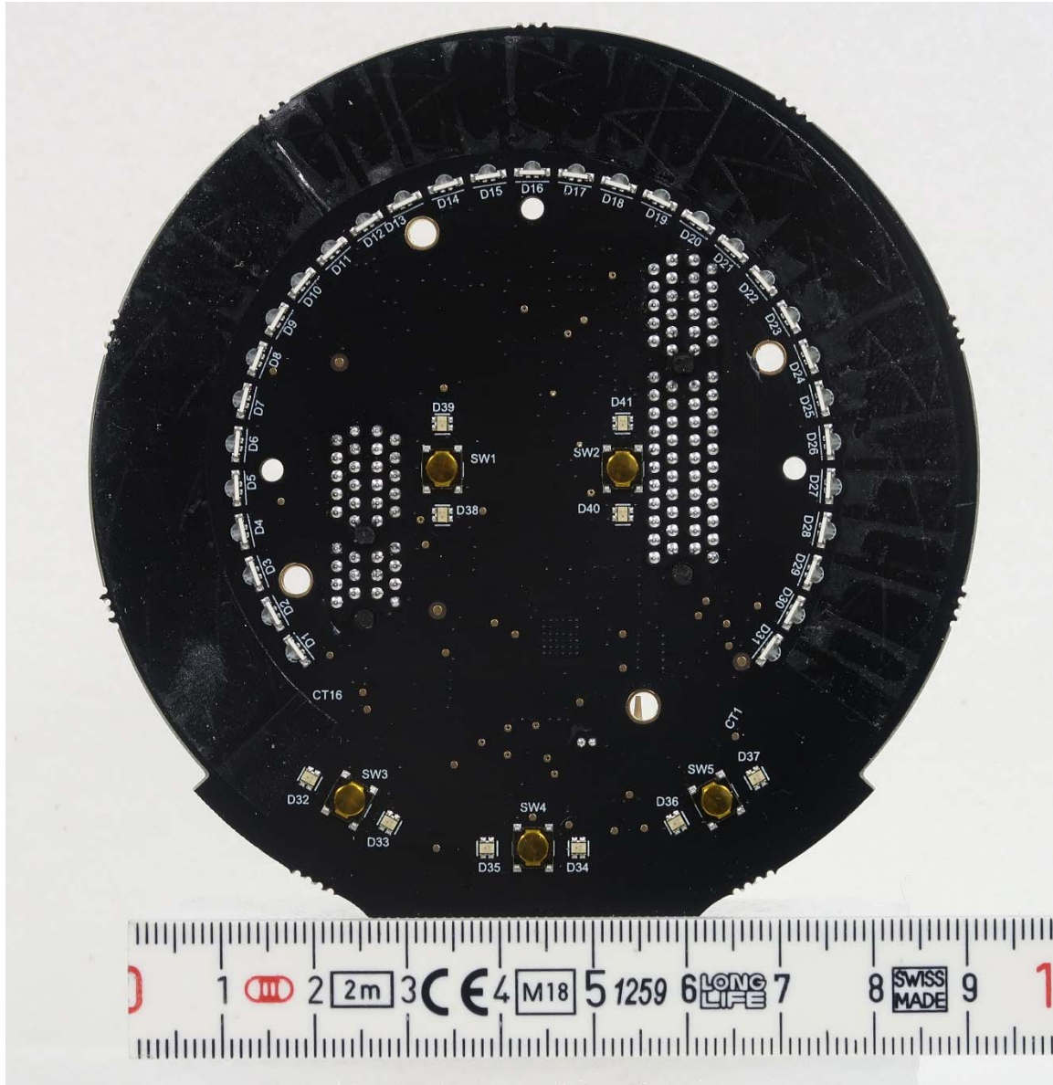
Tonos HA – 426 UI Module side 1
