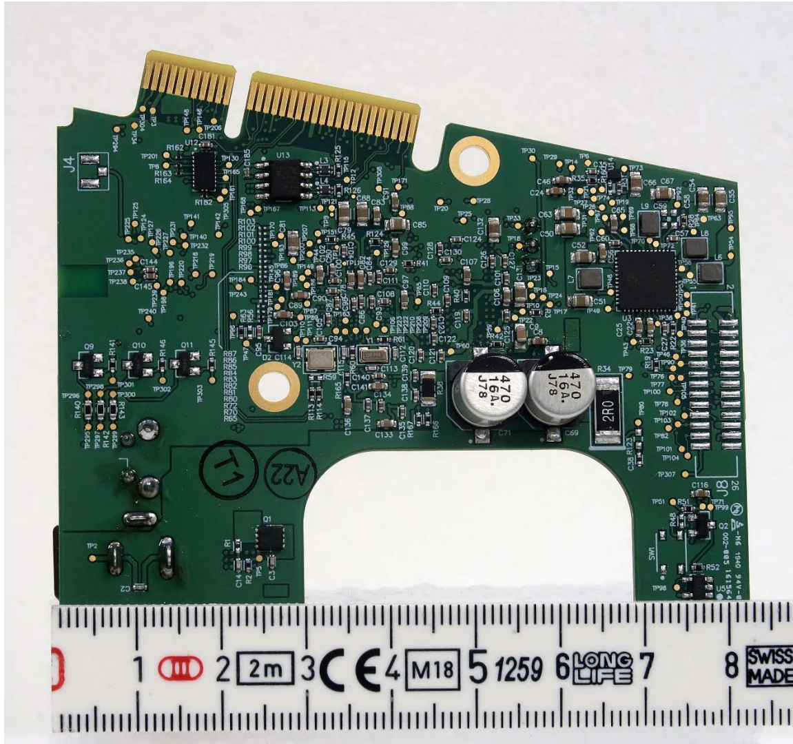
Tonos HA – 414 CPU Module side 1
