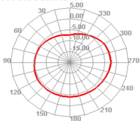
1990.000MHz H
