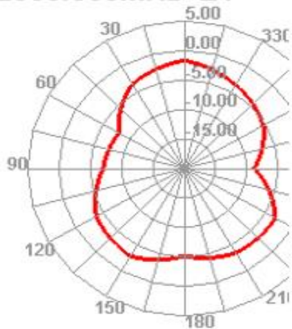
2550.000MHz E1
