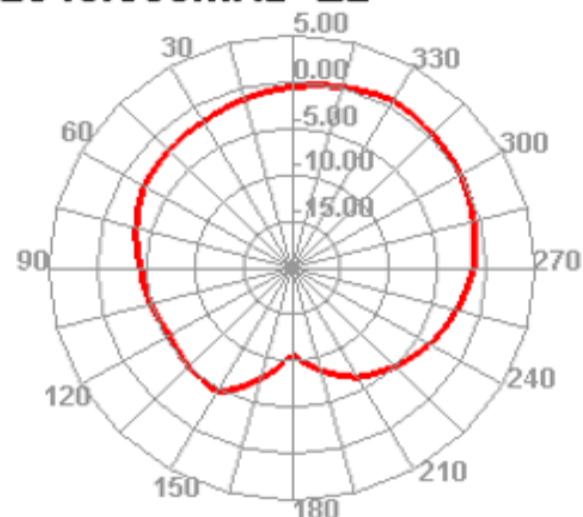
2340.000MHz E2
