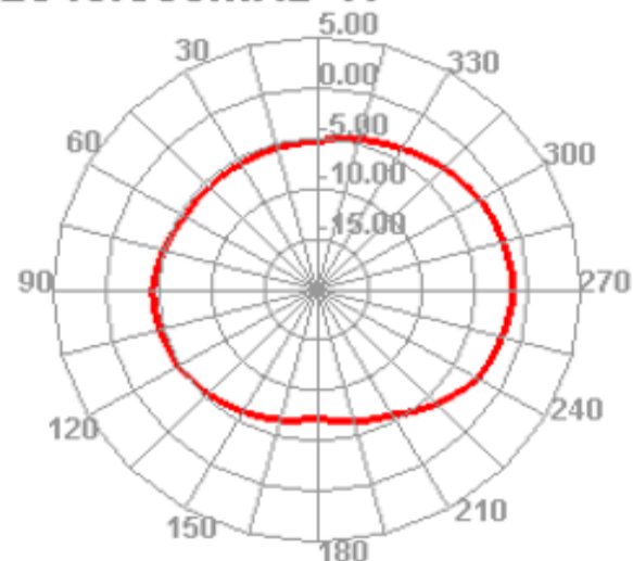
2340.000MHz H
