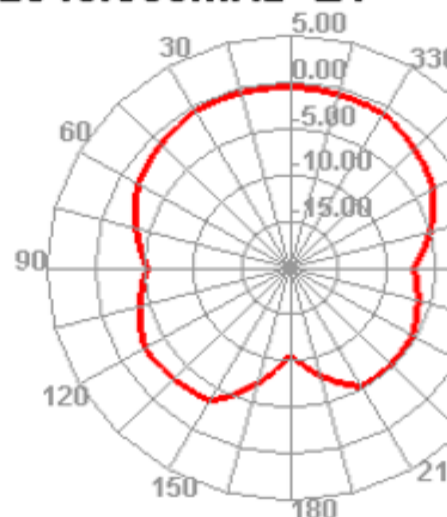
2340.000MHz E1
