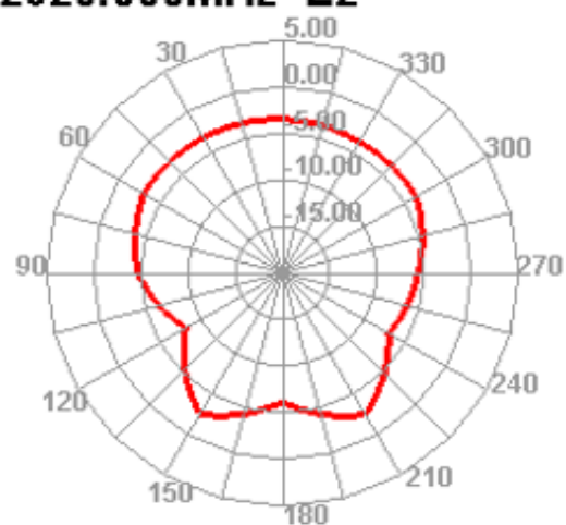
2620.000MHz E2
