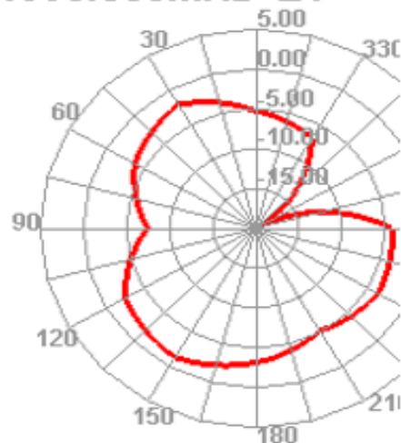
1990.000MHz E1
