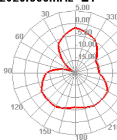
2620.000MHz E1
