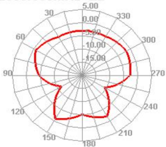
2550.000MHz E2
