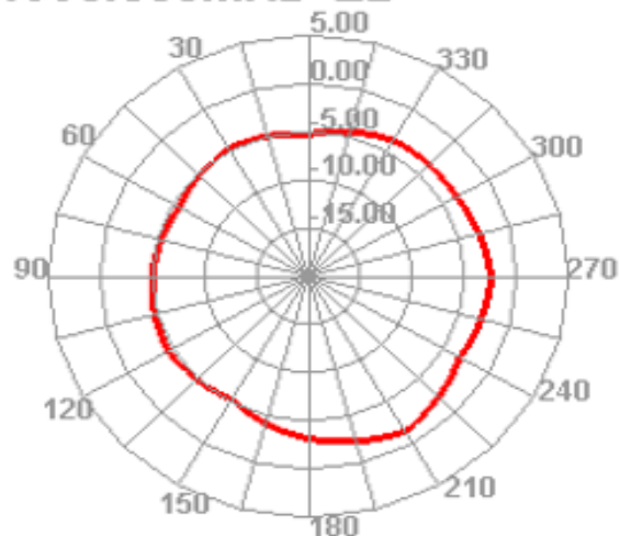
1990.000MHz E2
