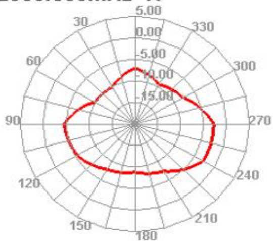
2550.000MHz H
