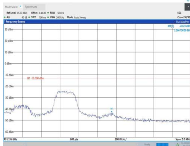
Band40-5MHz-QPSK-39225-1RB#24
