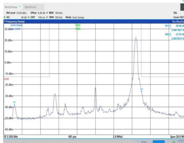
Band40-10MHz-QPSK-39200-50RB#0
