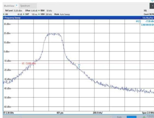
Band40-5MHz-QPSK-39225-25RB#0
