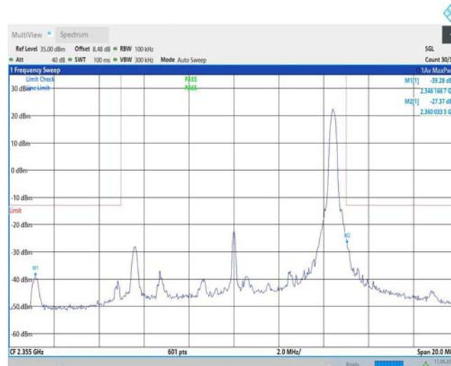
Band40-10MHz-QPSK-39200-50RB#0
