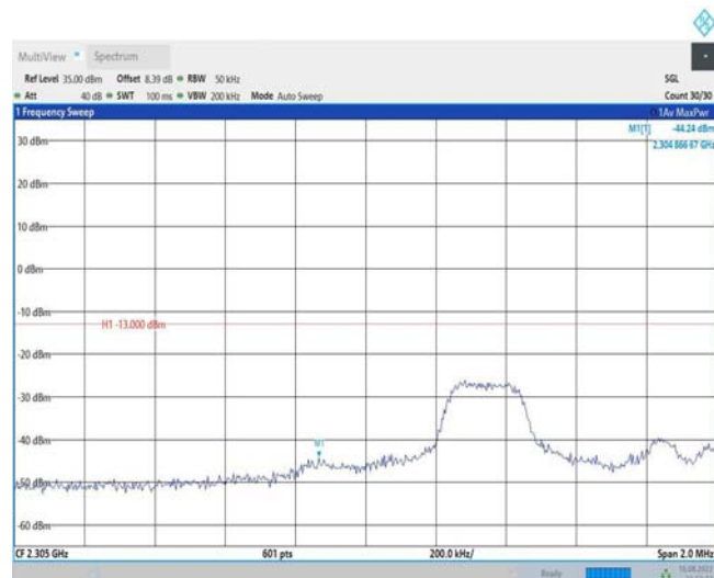
Band40-5MHz-QPSK-38725-25RB#0
