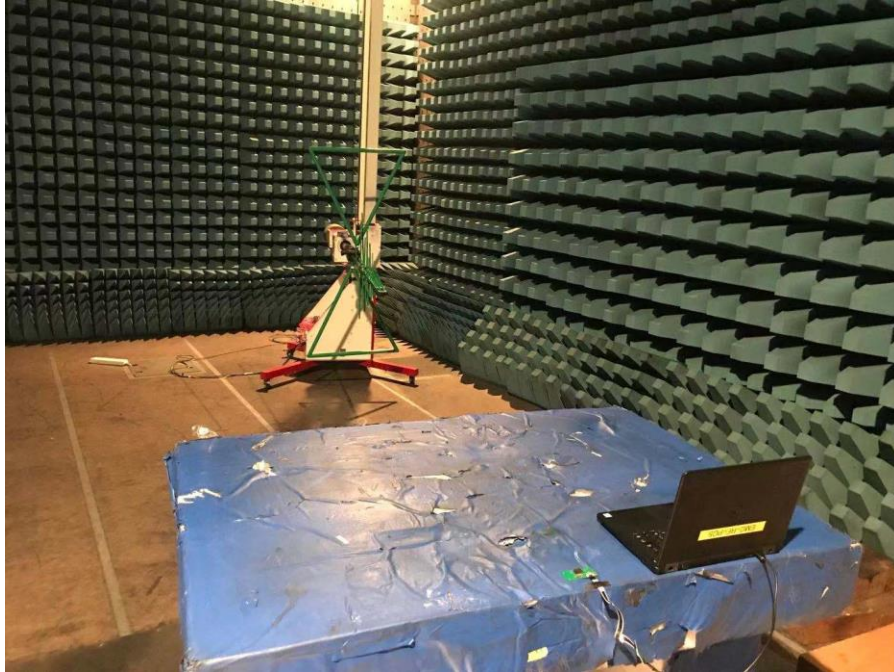
30-1000MHz
