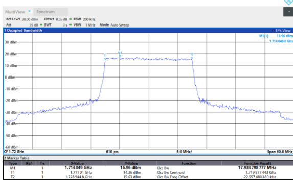
Band66-20MHz-QPSK-132572-100RB#0
