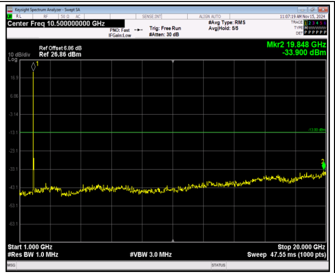
Band2-20MHz-16QAM-18900-1RB#0-Range2:1000~20000MHz
