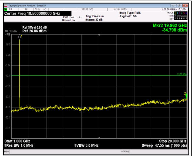
Band4-1.4MHz-QPSK-19957-1RB#0-Range2:1000~2 0000MHz
