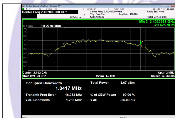
BLE 1M_Channel 0
