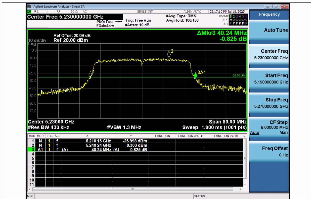
11AC40MIMO-Ant1-5230
