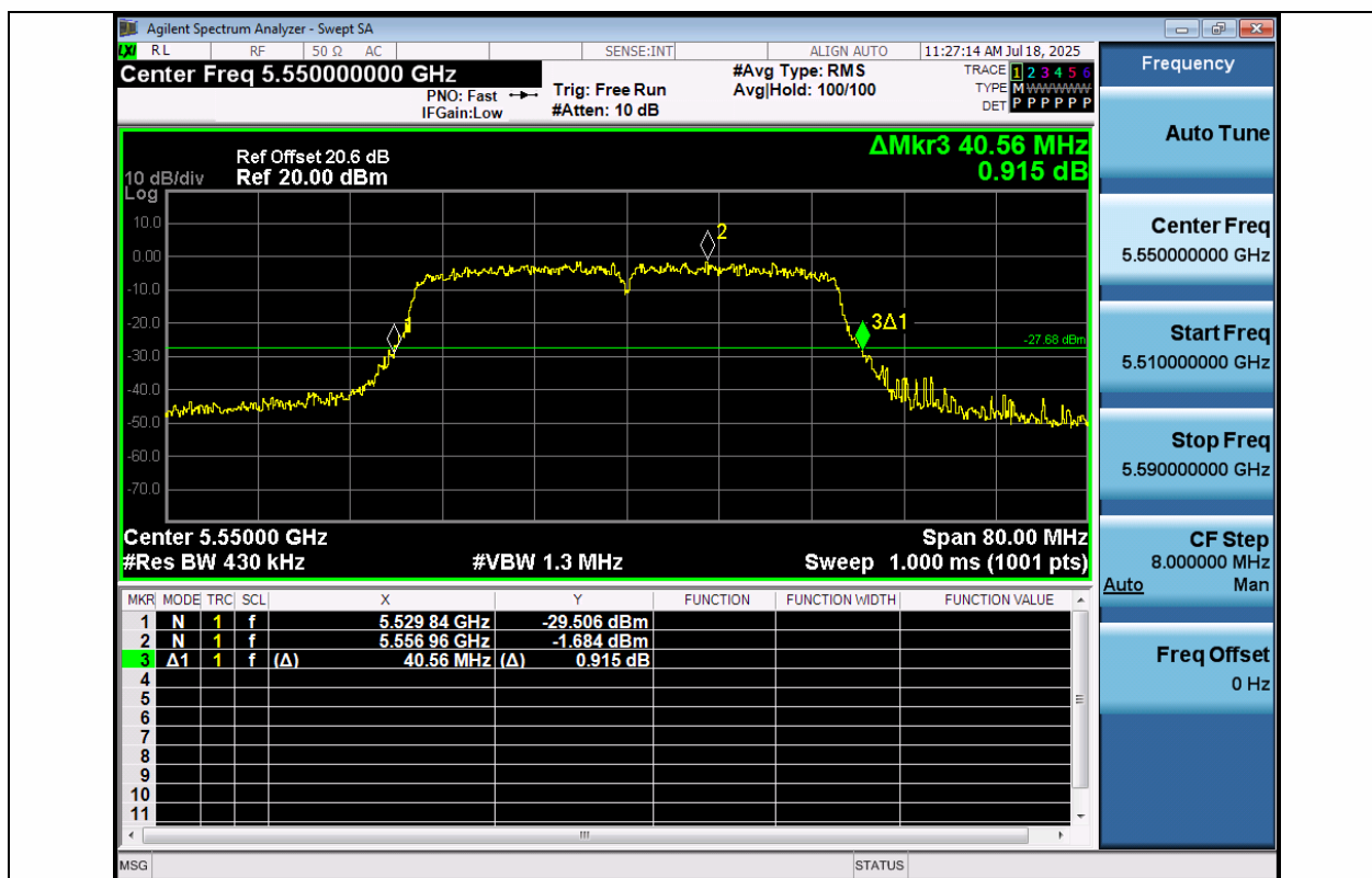
11N40MIMO-Ant1-5550
