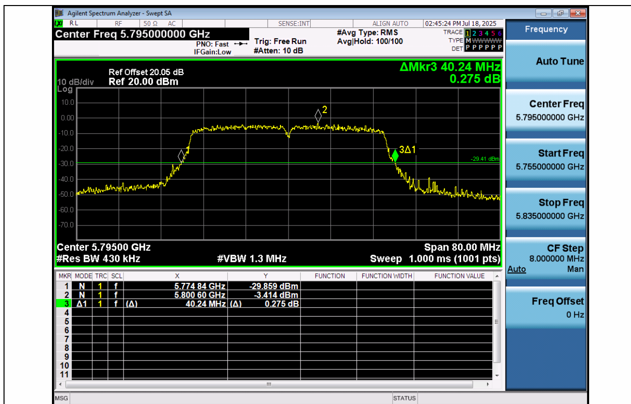
11AC40MIMO-Ant1-5795
