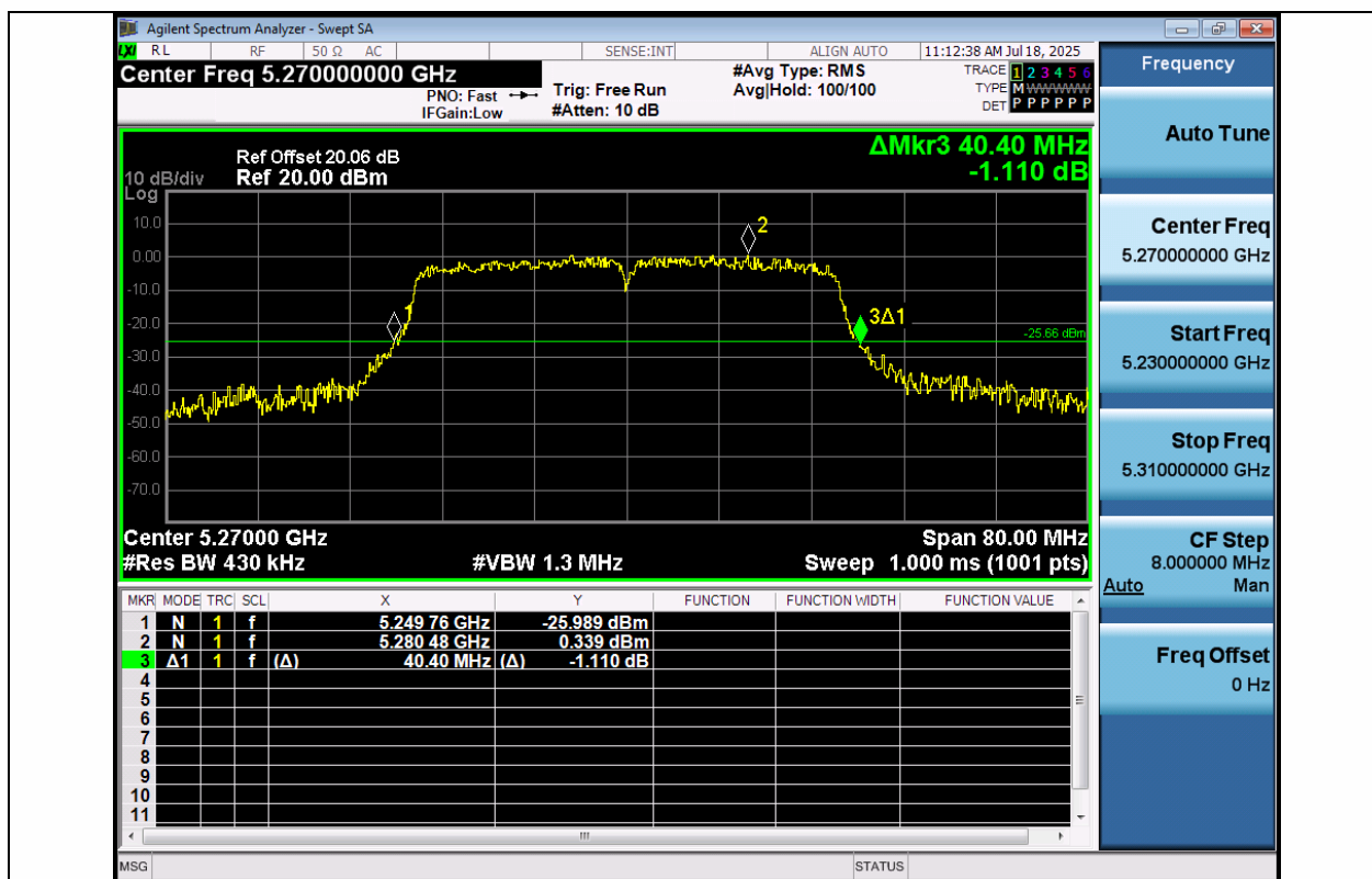
11N40MIMO-Ant1-5270
