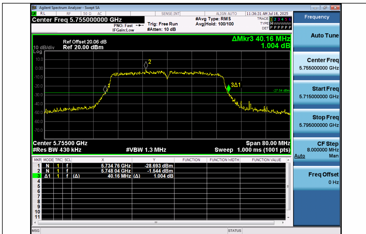
11N40MIMO-Ant1-5755
