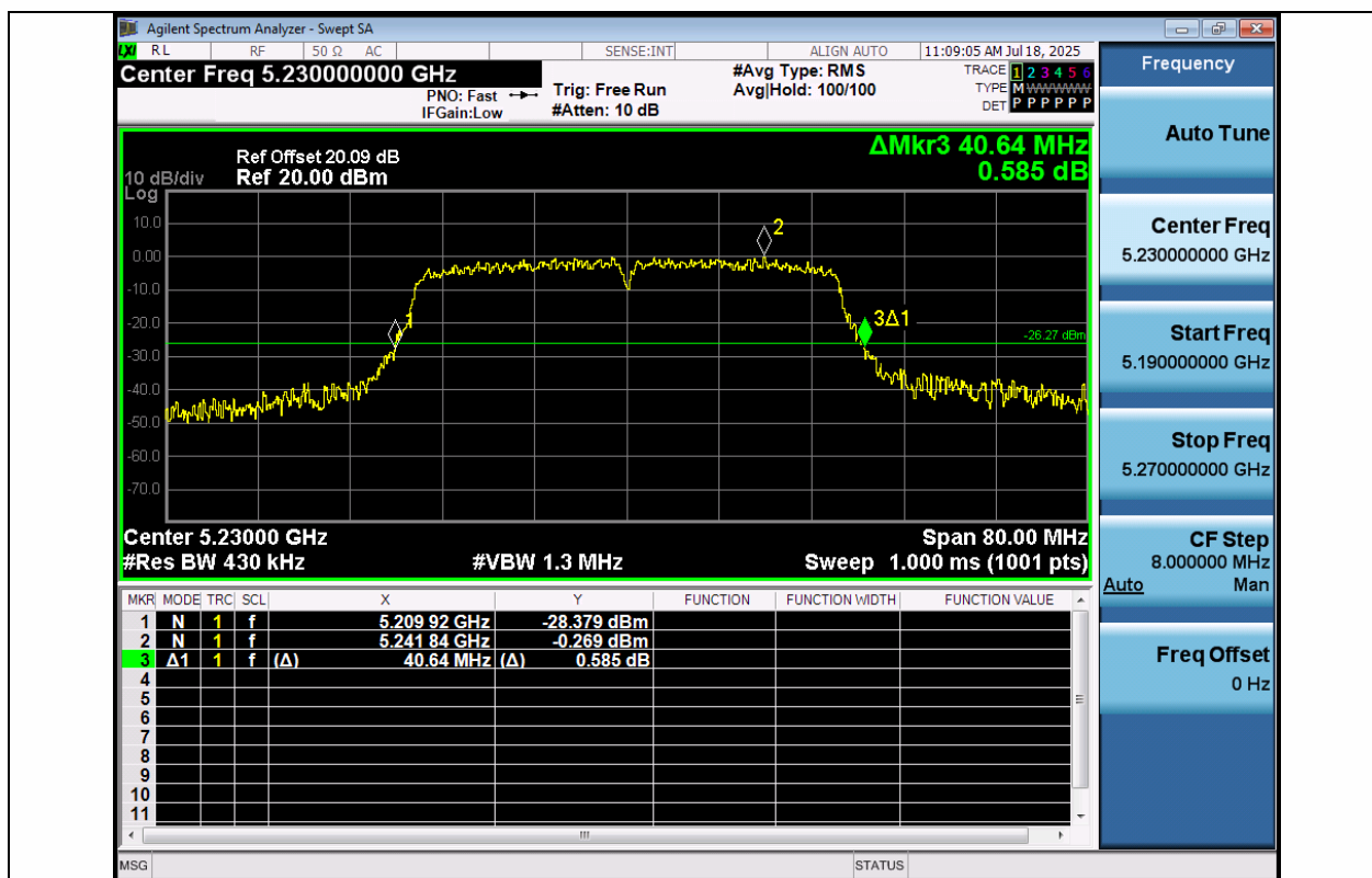
11N40MIMO-Ant1-5230
