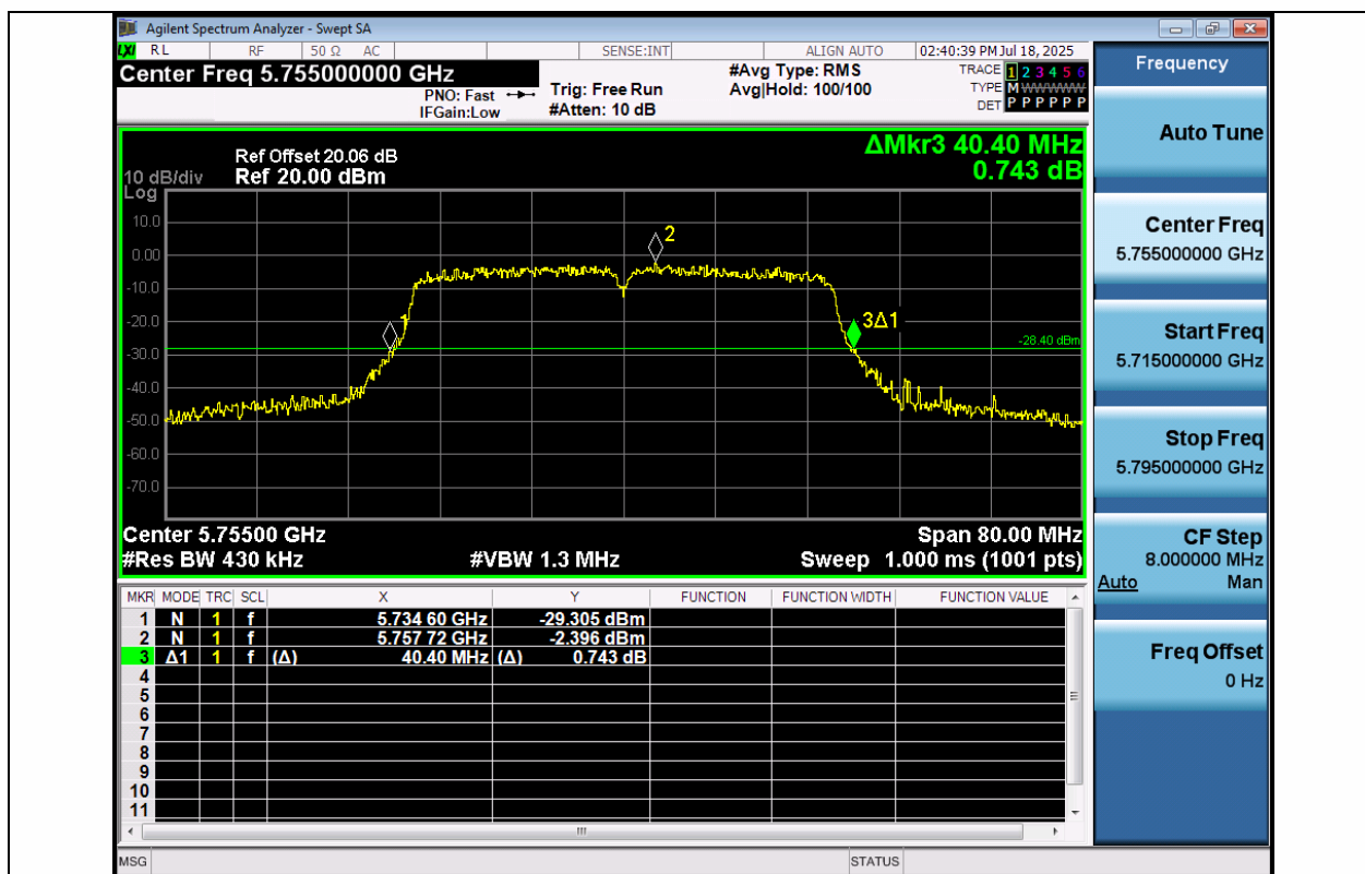
11AC40MIMO-Ant1-5755
