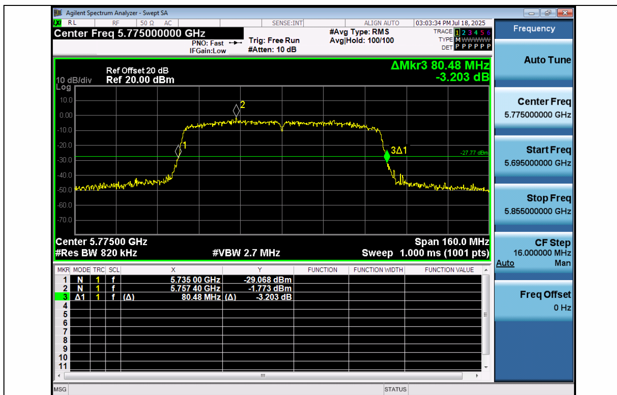
11AC80MIMO-Ant1-5775
