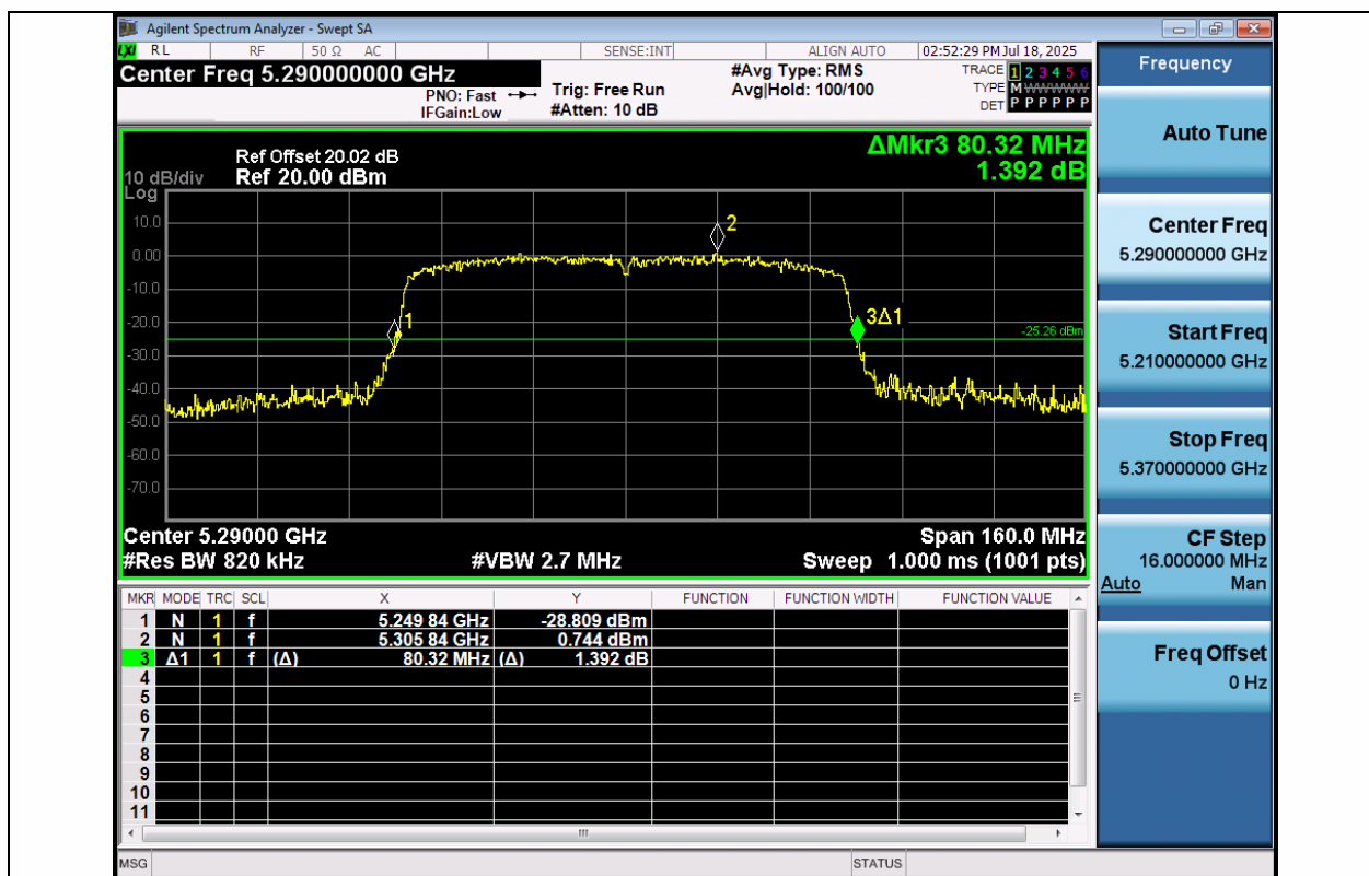
11AC80MIMO-Ant1-5290
