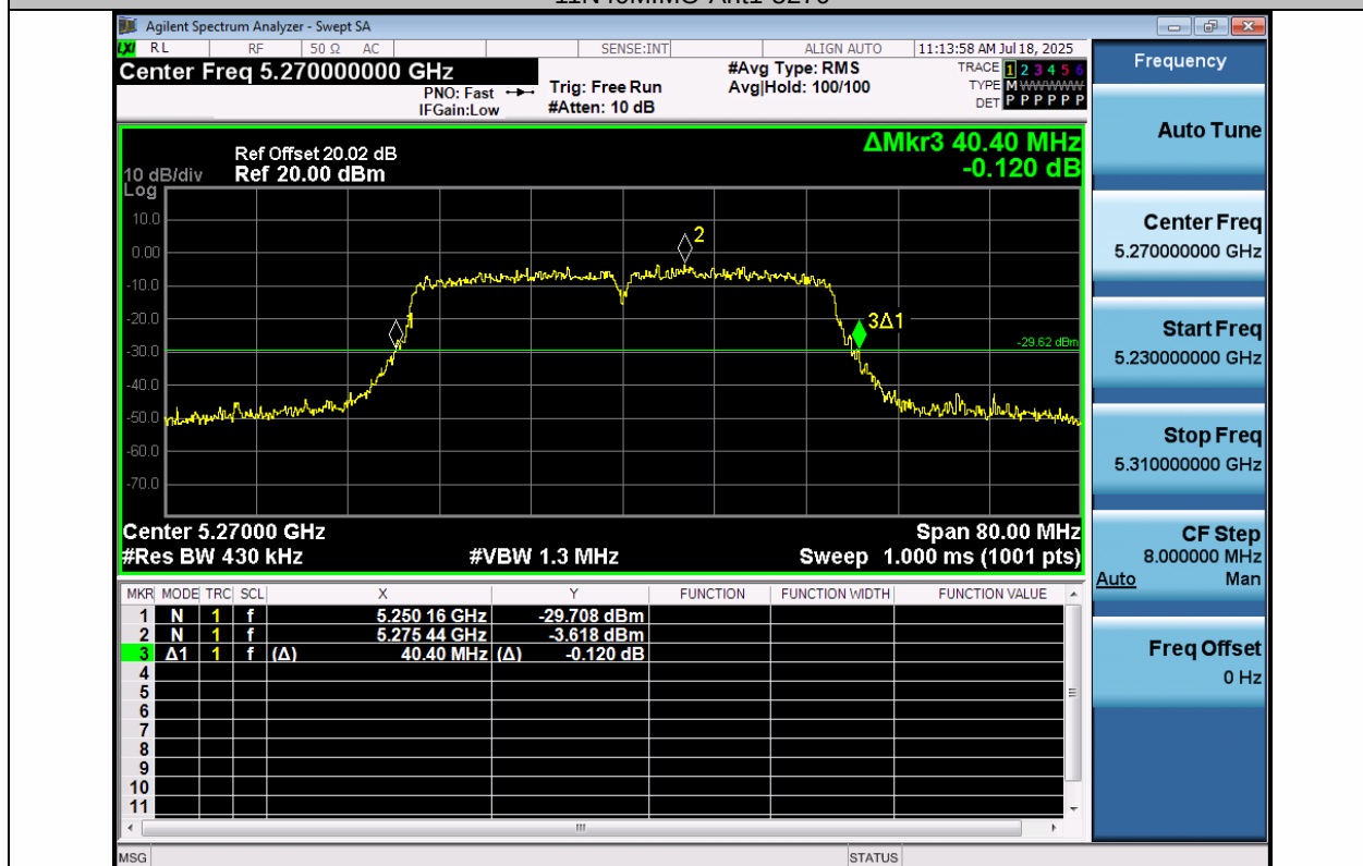
11N40MIMO-Ant2-5270
