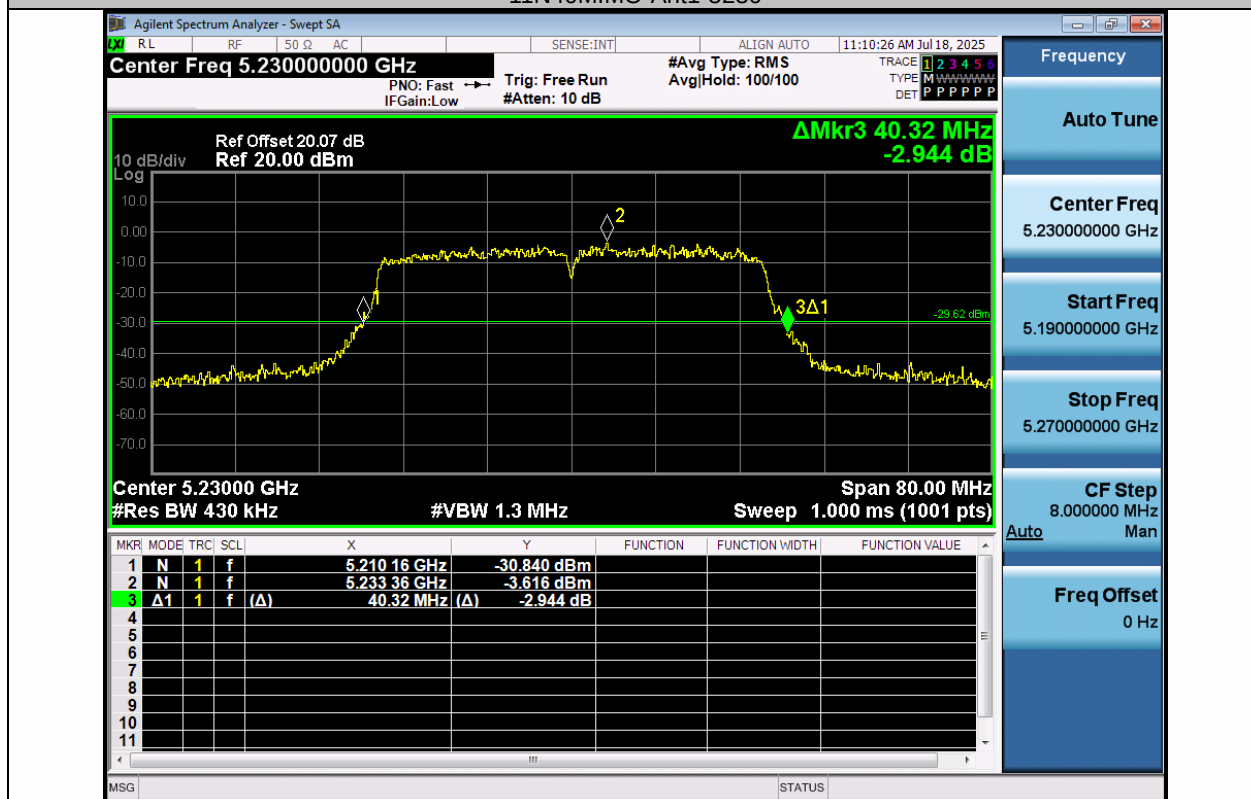
11N40MIMO-Ant2-5230
