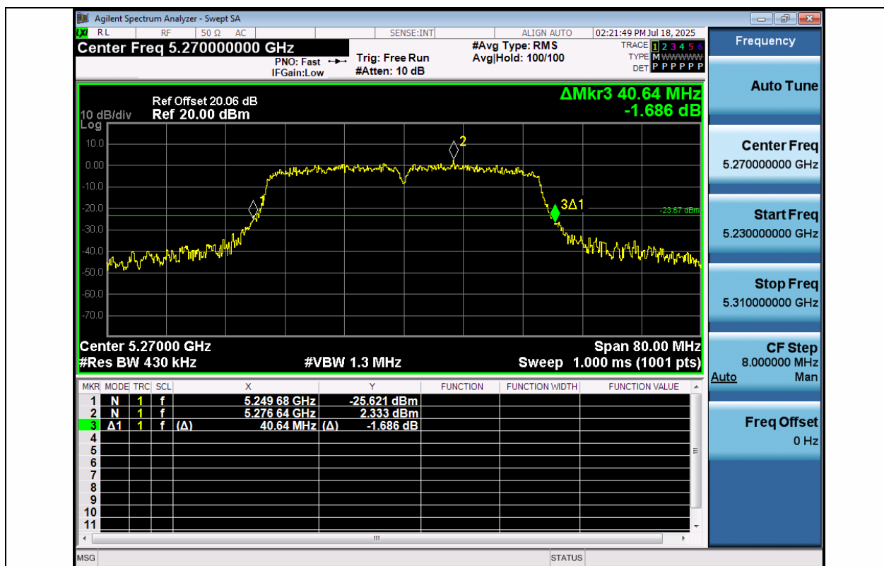
11AC40MIMO-Ant1-5270
