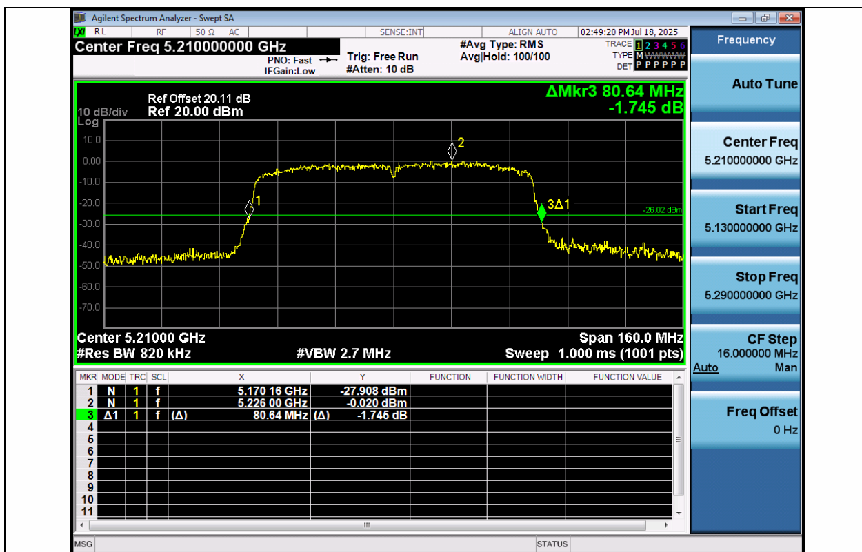
11AC80MIMO-Ant1-5210
