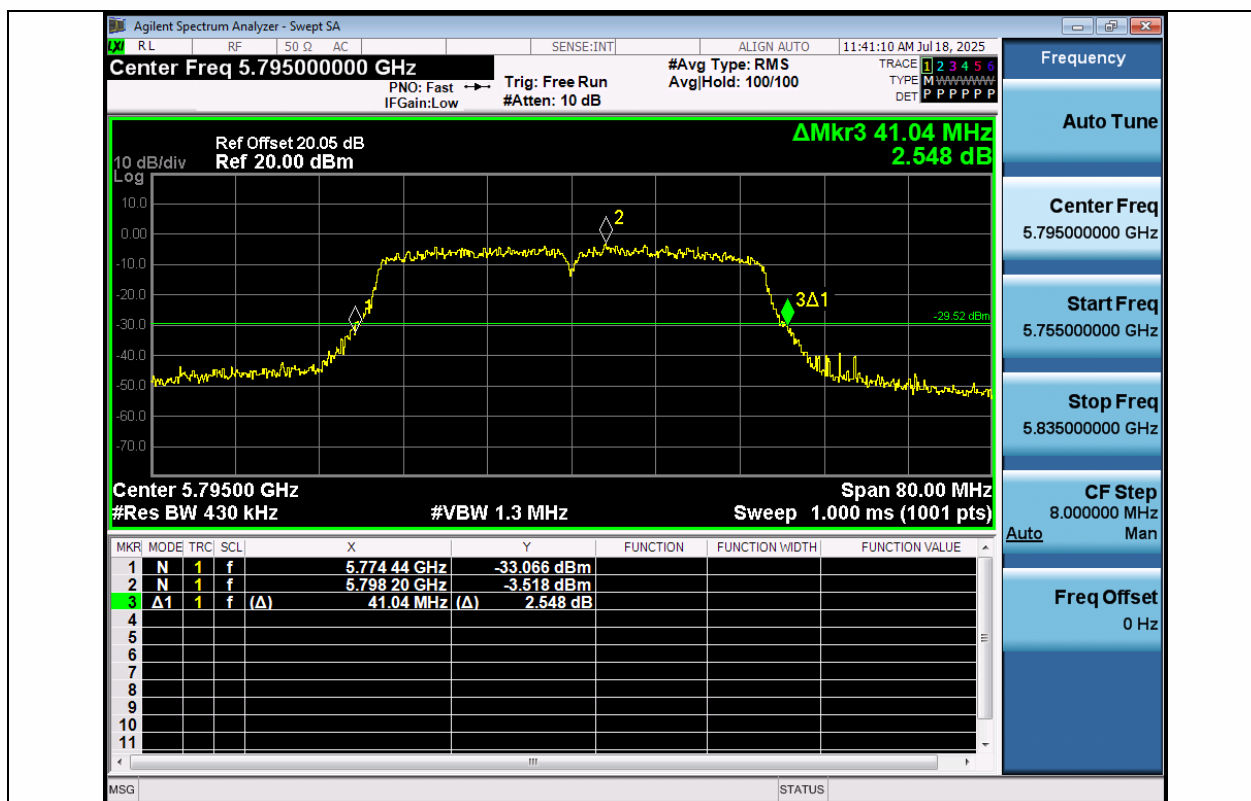
11N40MIMO-Ant1-5795
