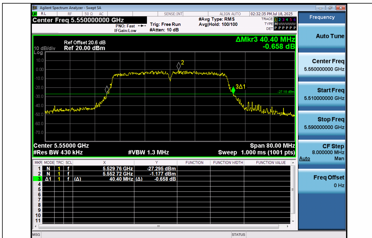
11AC40MIMO-Ant1-5550
