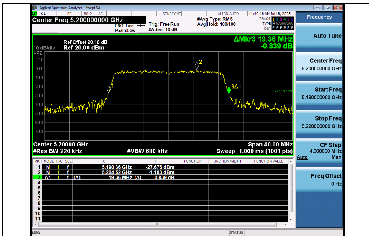
11AC20MIMO-Ant1-5200
