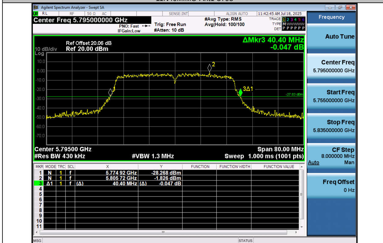
11N40MIMO-Ant2-5795
