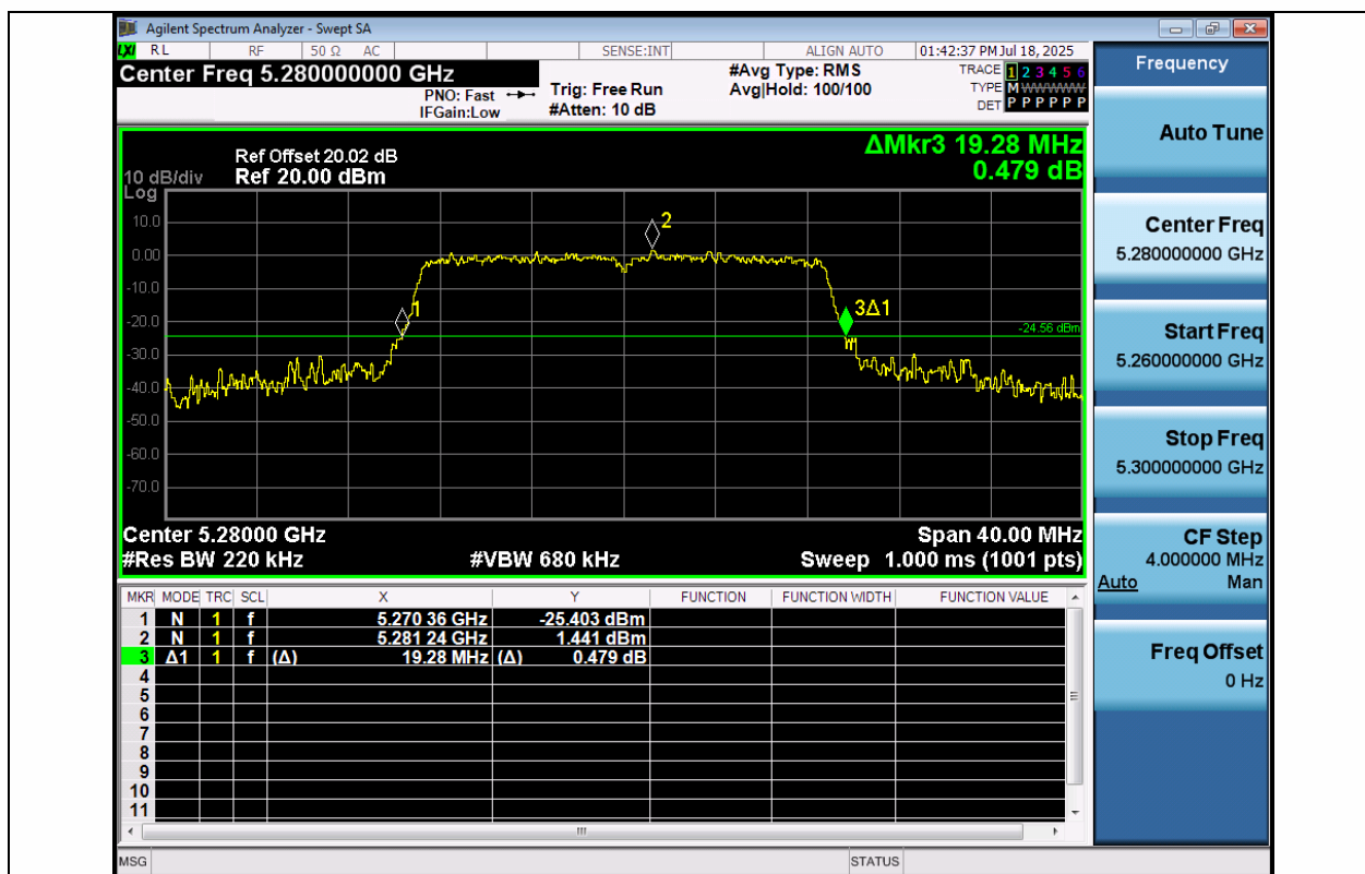
11AC20MIMO-Ant1-5280
