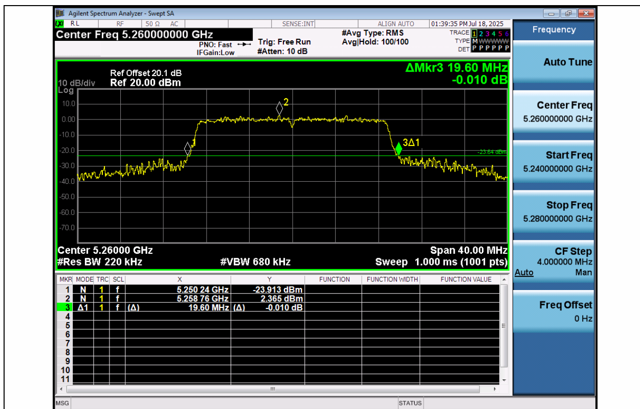
11AC20MIMO-Ant1-5260
