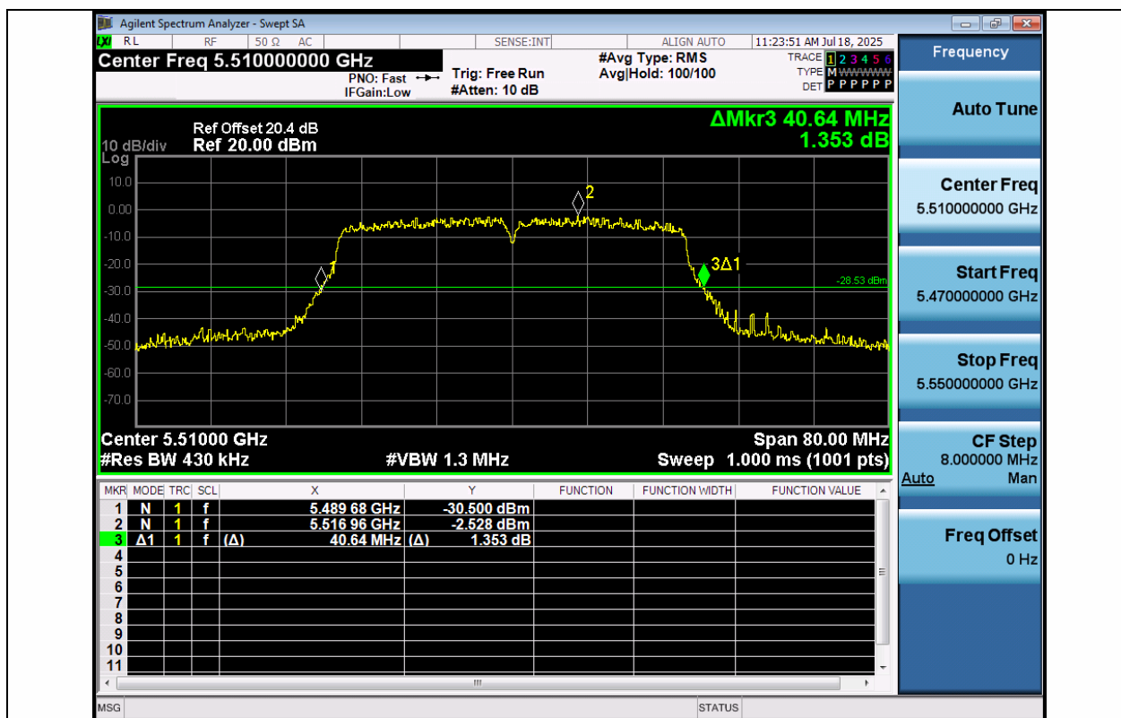
11N40MIMO-Ant1-5510
