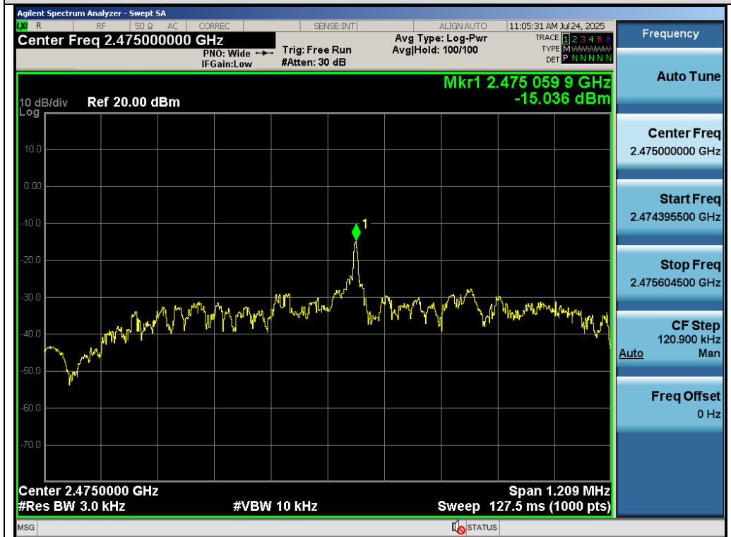
Test_Graph_GFSK_ANT1_2475_PSD
