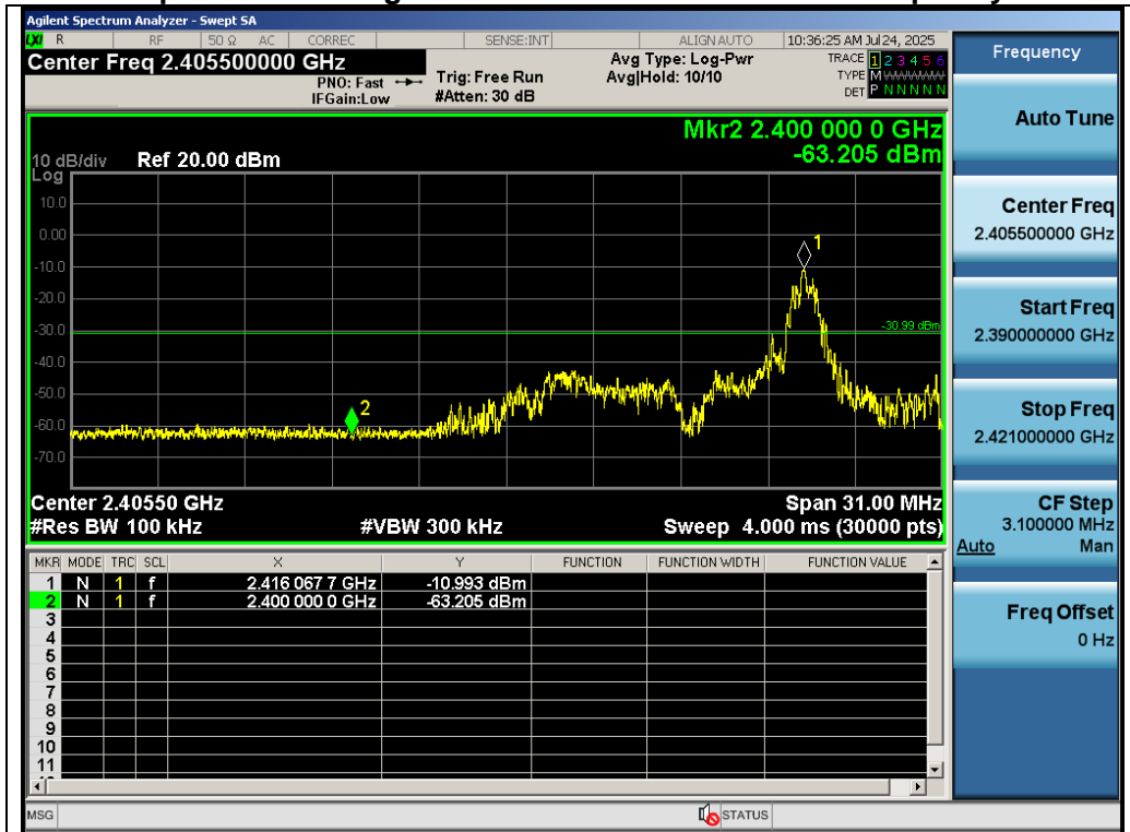
Test_Graph_GFSK_ANT1_2416_Lower Band Edge Emissions
