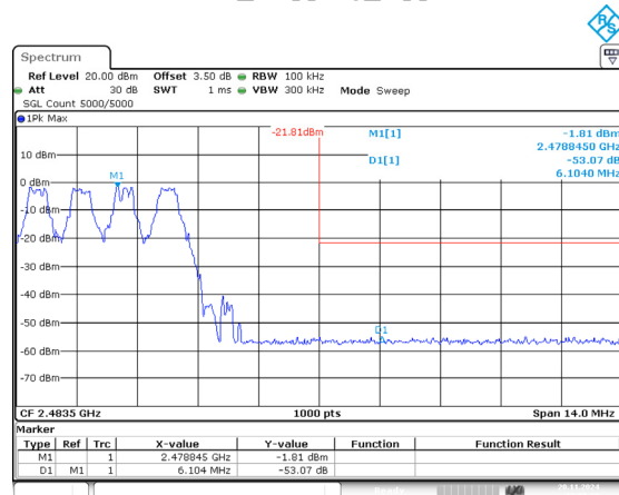
DH1_Hopping_Upper
