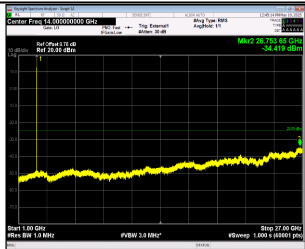
41-41-5MHz-20MHz-QPSK-QPSK-41373-41490-1RB#0-1RB#99-1000~27000MHz-PASS
