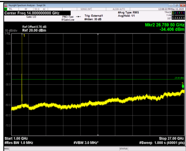
41-41-20MHz-10MHz-QPSK-QPSK-40571-40715-100RB#0 -50RB#0-1000~27000MHz-PASS
