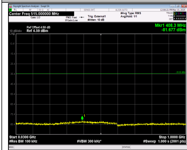
41-41-20MHz-10MHz-QPSK-QPSK-40571-40715-1RB#0 -1RB#49-30~1000MHz-PASS
