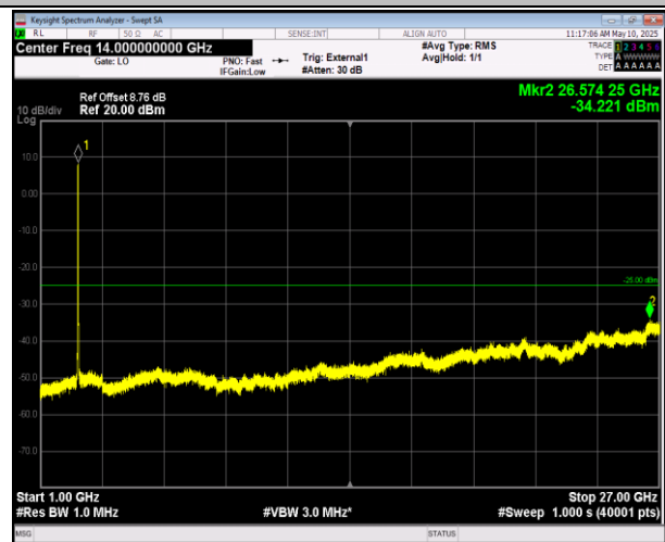
41-41-20MHz-5MHz-QPSK-QPSK-41440-41557-1RB#0-ORB#0-1000~27000MHz-PASS
