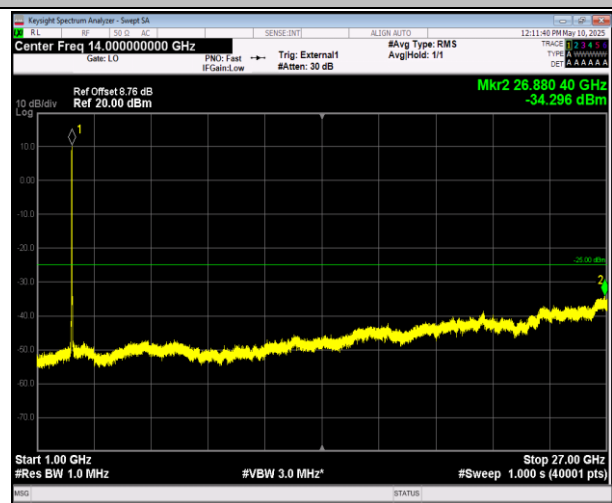
41-41-20MHz-10MHz-16QAM-16QAM-40571-40715-1RB#0 -0RB#0-1000~27000MHz-PASS
