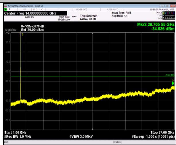
41-41-20MHz-5MHz-QPSK-QPSK-40595-40712-1RB#0-01RB#24-1000~27000MHz-PASS
