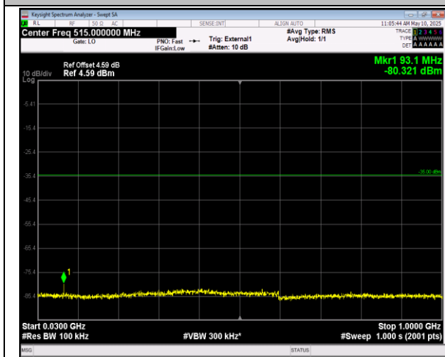
41-41-20MHz-5MHz-QPSK-QPSK-39750-39867-100RB# 0-25RB#0-30~1000MHz-PASS
