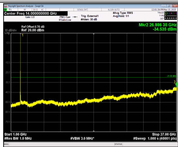
41-41-20MHz-10MHz-QPSK-QPSK-39750-39894-100RB#0 -50RB#0-1000~27000MHz-PASS
