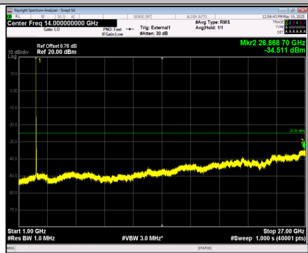
41-41-20MHz-10MHz-QPSK-QPSK-40571-40715-1RB#0-1 RB#49-1000~27000MHz-PASS
