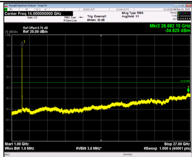
41-41-20MHz-5MHz-QPSK-QPSK-40595-40712-1RB#0-0RB#0-1000~27000MHz-PASS
