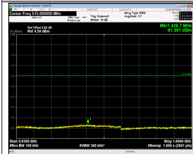
41-41-20MHz-10MHz-QPSK-QPSK-40571-40715-1RB#9 9-0RB#0-30~1000MHz-PASS
