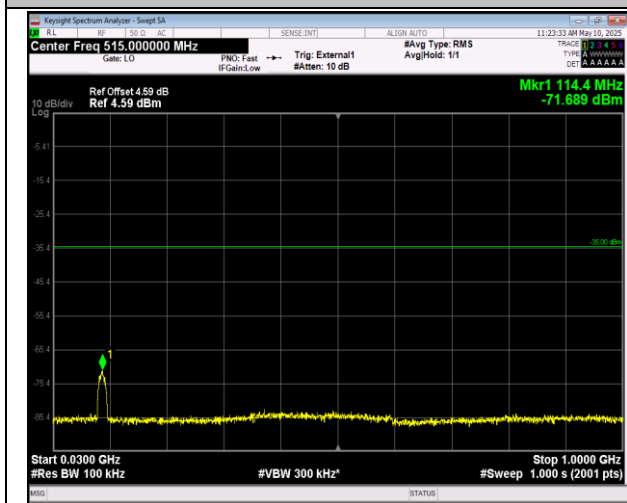
41-41-20MHz-10MHz-QPSK-QPSK-39750-39894-1RB#0 -0RB#0-30~1000MHz-PASS
