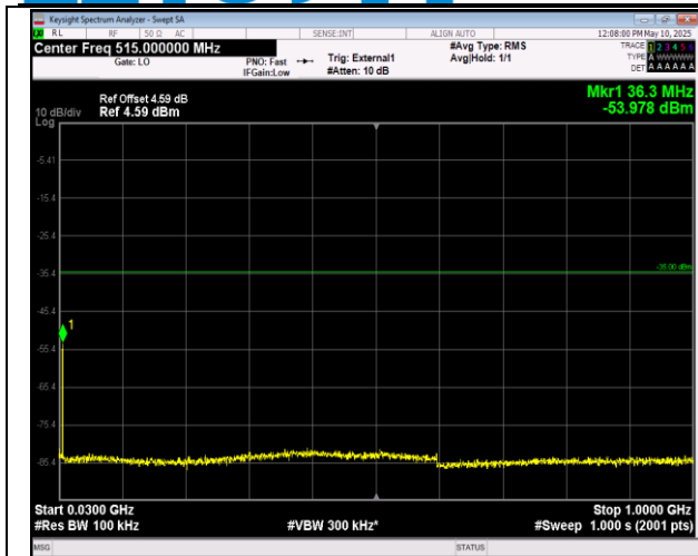
41-41-20MHz-10MHz-QPSK-QPSK-40571-40715-100RB #0-50RB#0-30~1000MHz-PASS
