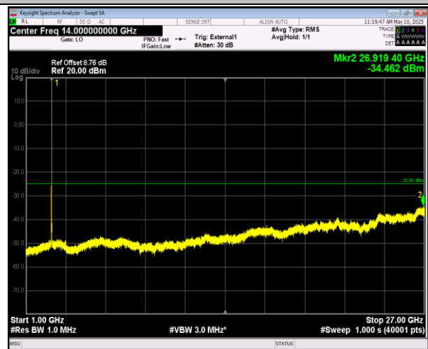
41-41-20MHz-5MHz-QPSK-QPSK-41440-41557-100RB#0-25RB#0-1000~27000MHz-PASS
