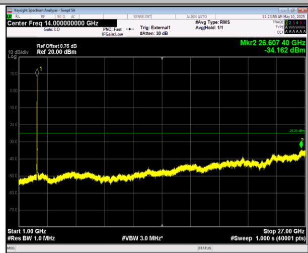
41-41-20MHz-10MHz-QPSK-QPSK-39750-39894-1RB#0-0 RB#0-1000~27000MHz-PASS
