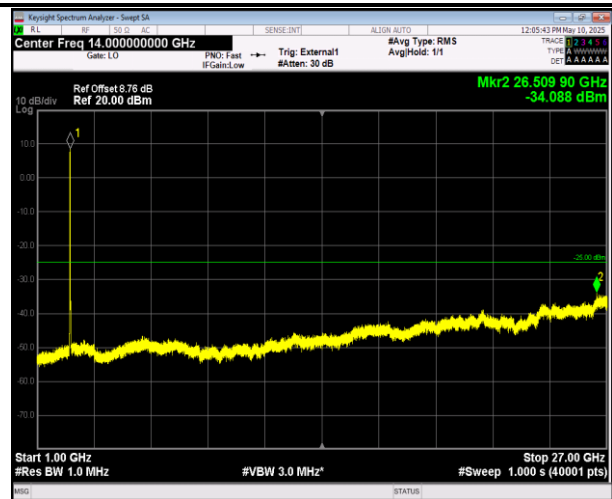
41-41-20MHz-10MHz-QPSK-QPSK-40571-40715-1RB#0-0 RB#0-1000~27000MHz-PASS
