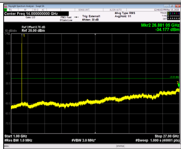
41-41-5MHz-20MHz-16QAM-16QAM-41373-41490-1RB#0- 1RB#99-1000~27000MHz-PASS
