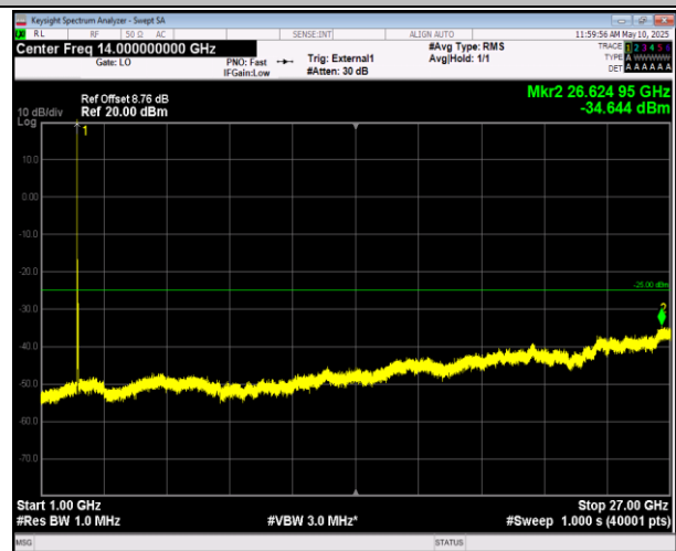
41-41-20MHz-10MHz-QPSK-QPSK-39750-39894-1RB#0-1 RB#49-1000~27000MHz-PASS
