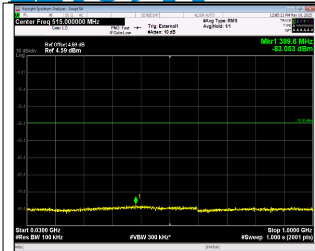
41-41-20MHz-10MHz-QPSK-QPSK-40571-40715-1RB#0 -0RB#0-30~1000MHz-PASS
