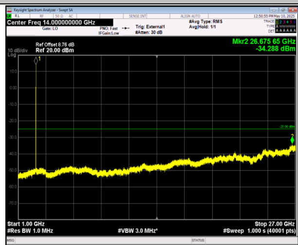
41-41-20MHz-5MHz-QPSK-QPSK-39750-39867-1RB#0-0R B#0-1000~27000MHz-PASS
