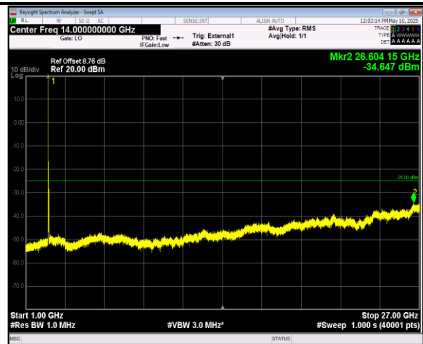
41-41-20MHz-10MHz-QPSK-QPSK-39750-39894-1RB#99- ORB#0-1000~27000MHz-PASS
