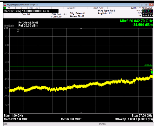
41-41-5MHz-20MHz-QPSK-QPSK-41373-41490-1RB#0-ORB#0-1000~27000MHz-PASS
