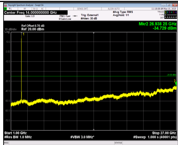
41-41-20MHz-5MHz-QPSK-QPSK-41440-41557-1RB#0-1RB#24-1000~27000MHz-PASS
