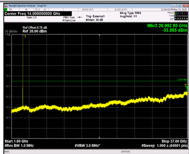
41-41-5MHz-20MHz-QPSK-QPSK-41373-41490-25RB#0-100RB#0-1000~27000MHz-PASS
