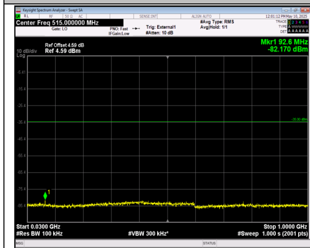
41-41-20MHz-10MHz-QPSK-QPSK-39750-39894-100RB #0-50RB#0-30~1000MHz-PASS
