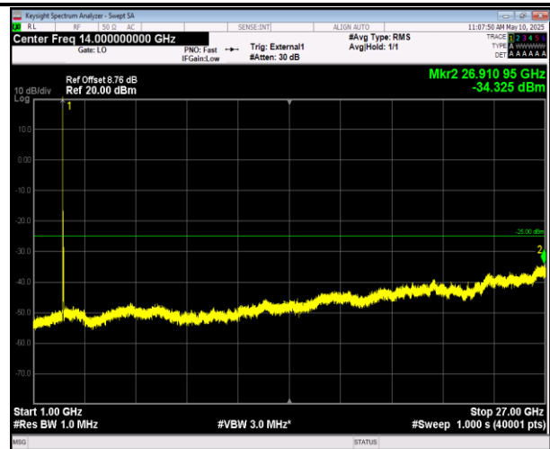
41-41-20MHz-5MHz-QPSK-QPSK-39750-39867-1RB#99-0 RB#0-1000~27000MHz-PASS
