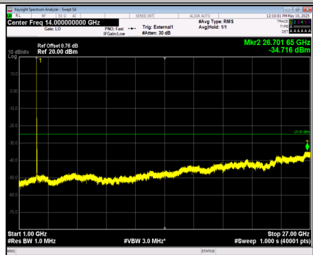
41-41-20MHz-10MHz-QPSK-QPSK-40571-40715-1RB#99- ORB#0-1000~27000MHz-PASS
