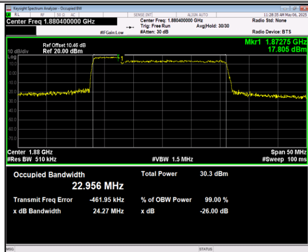
2-2-5MHz-20MHz-QPSK-QPSK-18983-19100-25RB#0-1 00RB#0-PASS
