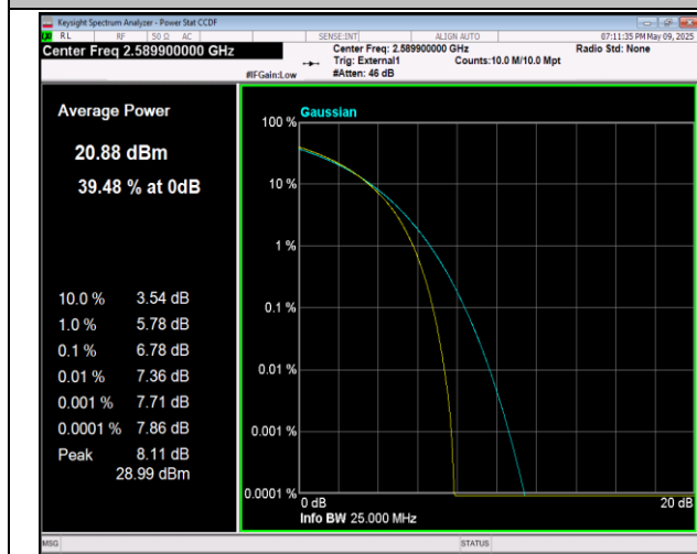
38-38-20MHz-20MHz-QPSK-QPSK-37901-38099-100RB# 0-100RB#0-PASS
