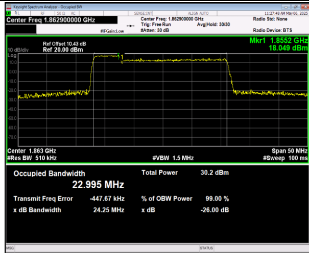
2-2-5MHz-20MHz-QPSK-QPSK-18808-18925-25RB#0-1 00RB#0-PASS
