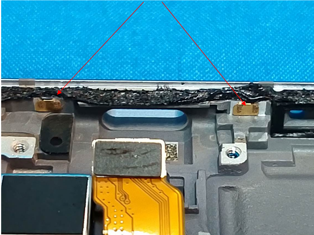
WWAN Antenna(ANT 0)
