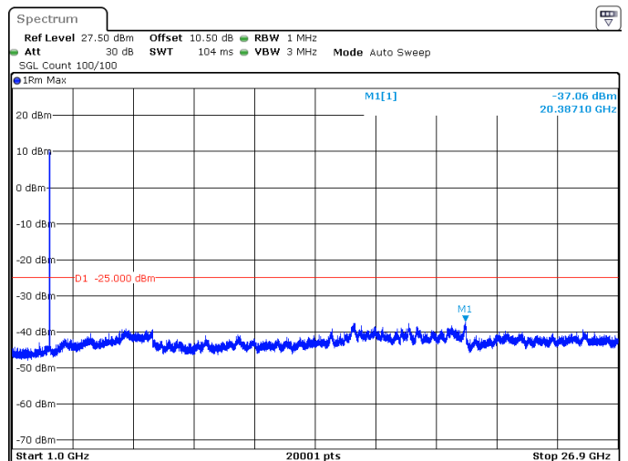
20MHz_15kHz_2593.005MHz_DFT-s-OFDM QPSK_RB100@0 -37.06 dBm
