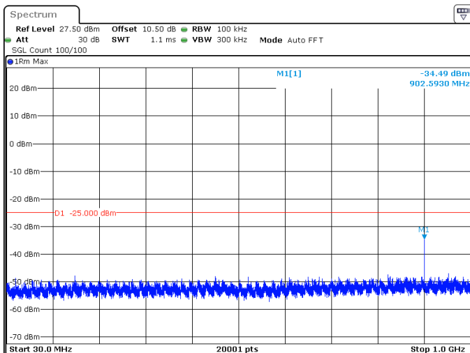
20MHz_15kHz_2593.005MHz_DFT-s-OFDM QPSK_RB100@0 -34.49 dBm
