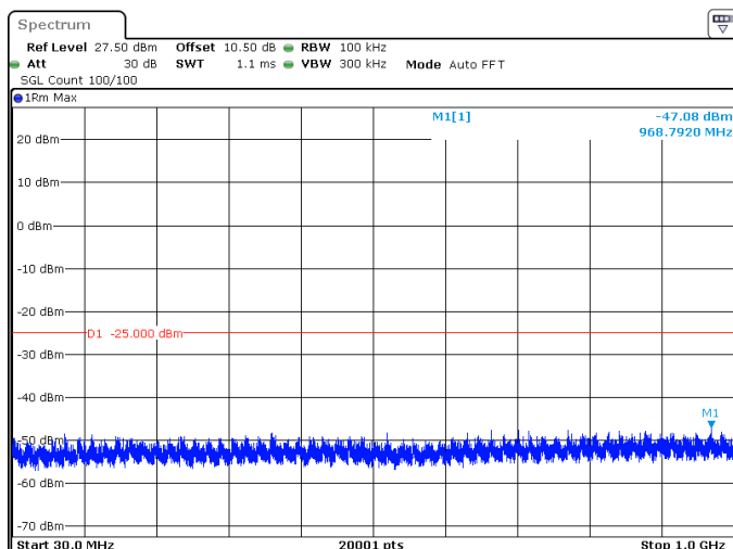
15MHz_30kHz_2682.48MHz_DFT-s-OFDM QPSK_RB36@0 -47.08 dBm
