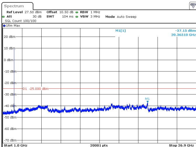
20MHz_30kHz_2506.02MHz_DFT-s-OFDM QPSK_RB50@0 -37.15 dBm
