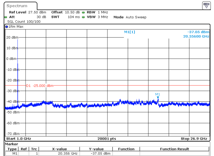
10MHz_30kHz_2592.99MHz_DFT-s-OFDM QPSK_RB1@0 -37.05 dBm
