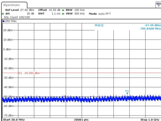
50MHz_15kHz_2593.005MHz_DFT-s-OFDM QPSK_RB270@0 -47.49 dBm
