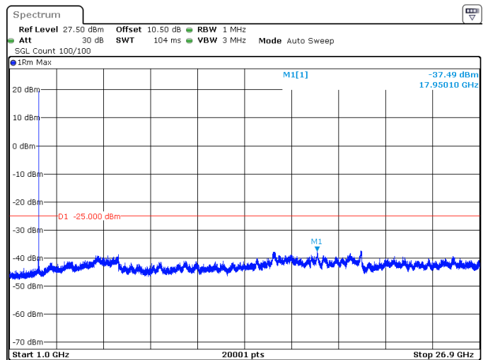
30MHz_15kHz_2593.005MHz_DFT-s-OFDM QPSK_RB1@159 -37.49 dBm
