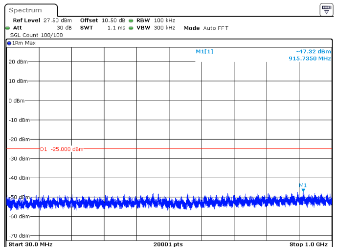
50MHz_15kHz_2521.005MHz_DFT-s-OFDM QPSK_RB270@0 -47.32 dBm
