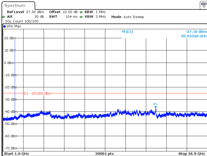
20MHz_30kHz_2506.02MHz_DFT-s-OFDM QPSK_RB1@50 -37.18 dBm
