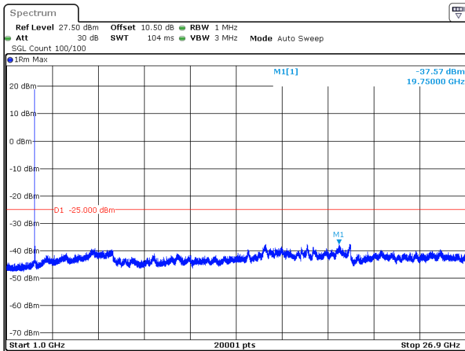
60MHz_30kHz_2592.99MHz_DFT-s-OFDM QPSK_RB1@0 -37.57 dBm
