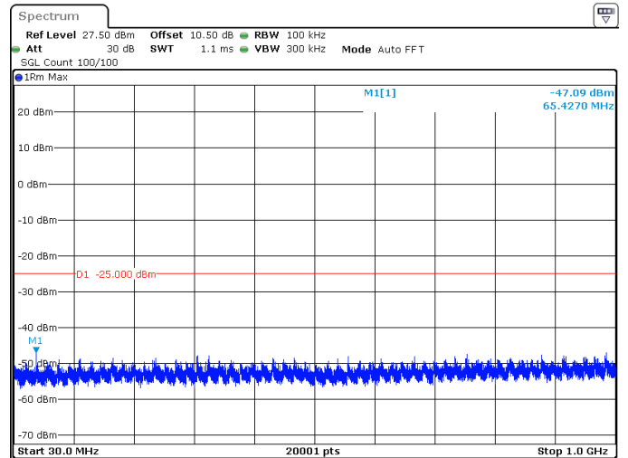
20MHz_30kHz_2506.02MHz_DFT-s-OFDM QPSK_RB1@50 -47.09 dBm
