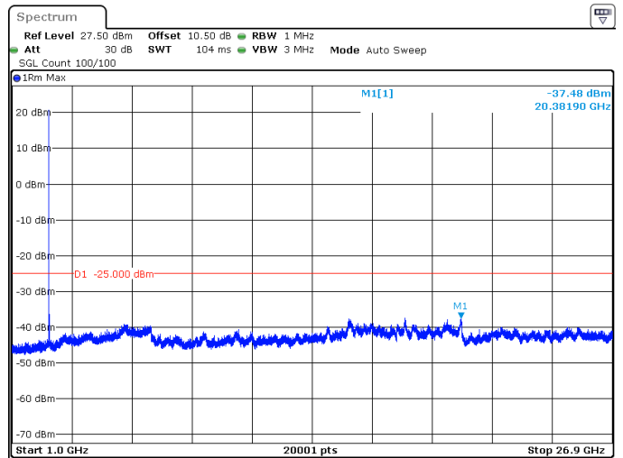
15MHz_15kHz_2593.005MHz_DFT-s-OFDM QPSK_RB1@0 -37.48 dBm
