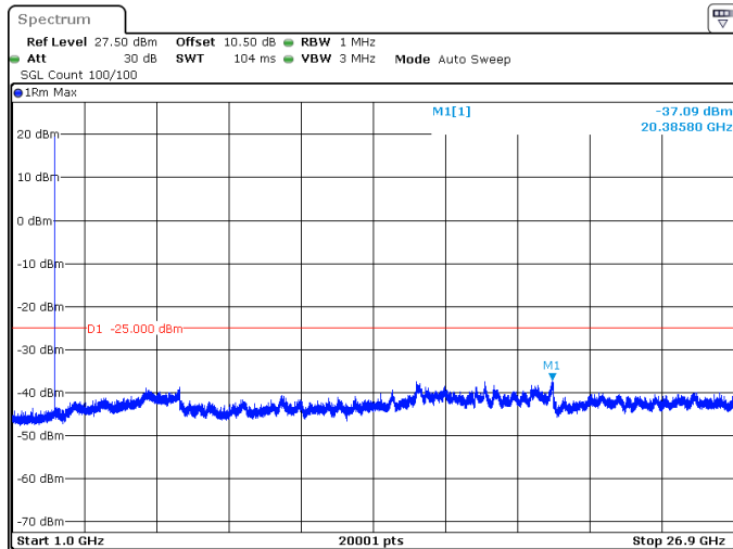
20MHz_15kHz_2506.005MHz_DFT-s-OFDM QPSK_RB1@105 -37.09 dBm
