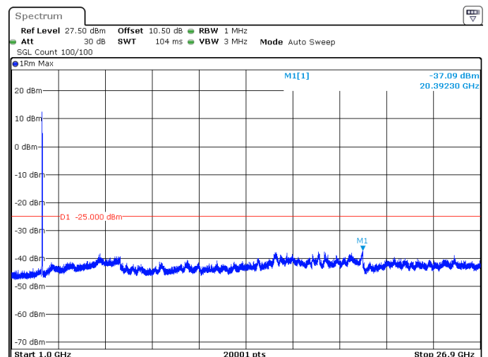
20MHz_30kHz_2679.99MHz_DFT-s-OFDM QPSK_RB50@0 -37.09 dBm
