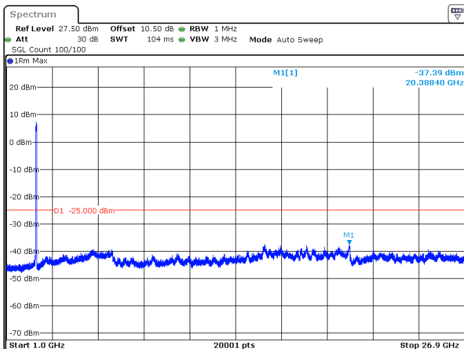
40MHz_15kHz_2670MHz_DFT-s-OFDM QPSK_RB216@0 -37.39 dBm
