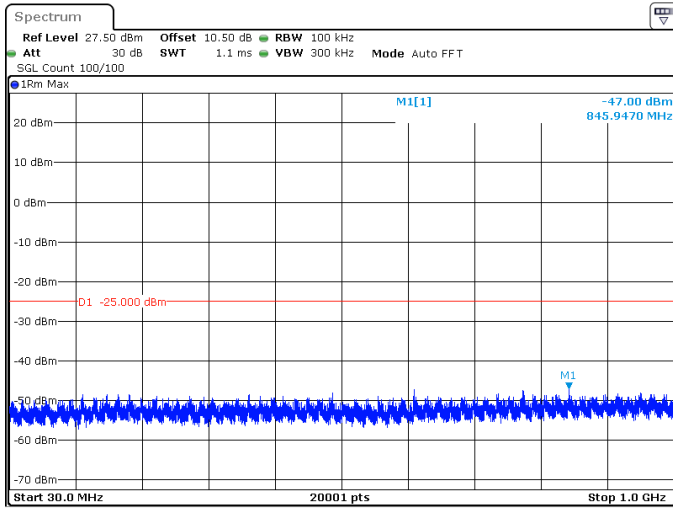
60MHz_30kHz_2526MHz_DFT-s-OFDM QPSK_RB1@0 -47.00 dBm
