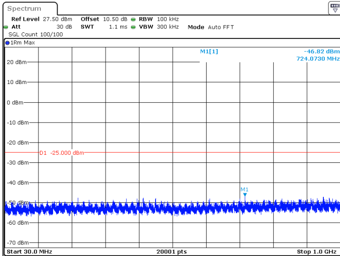
20MHz_30kHz_2506.02MHz_DFT-s-OFDM QPSK_RB1@0 -46.82 dBm
