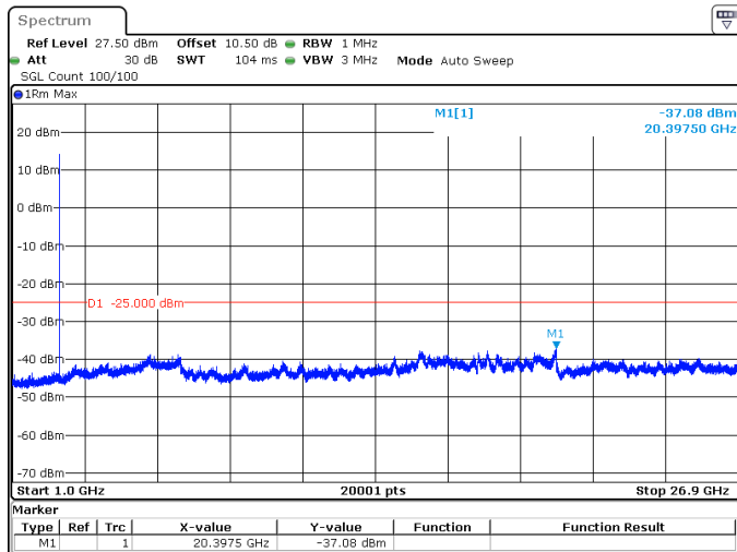
20MHz_30kHz_2679.99MHz_DFT-s-OFDM QPSK_RB1@0 -37.08 dBm
