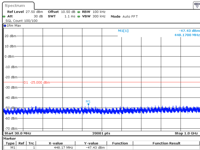
10MHz_30kHz_2592.99MHz_DFT-s-OFDM QPSK_RB1@0 -47.43 dBm
