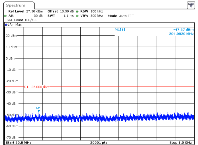
30MHz_30kHz_2511MHz_DFT-s-OFDM QPSK_RB1@0 -47.37 dBm
