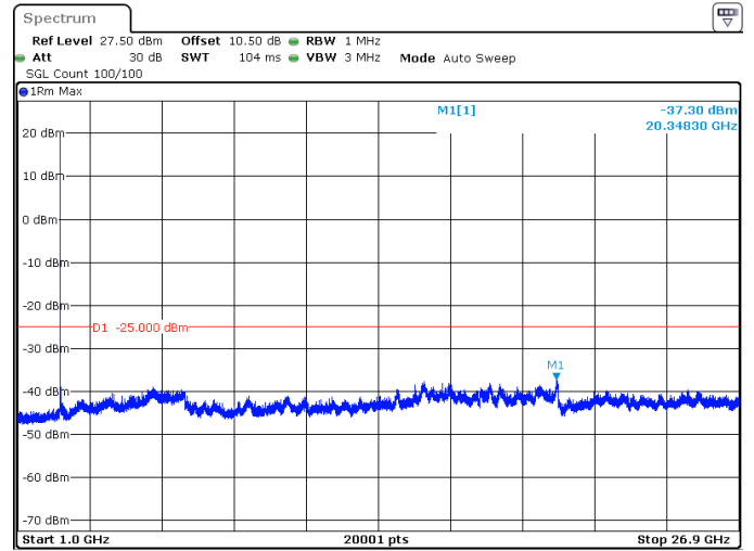
60MHz_30kHz_2526MHz_DFT-s-OFDM QPSK_RB1@0 -37.30 dBm
