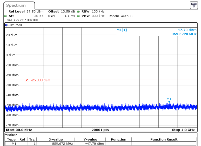
10MHz_30kHz_2685MHz_DFT-s-OFDM QPSK_RB1@0 -47.70 dBm
