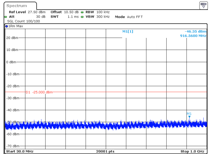
20MHz_30kHz_2592.99MHz_DFT-s-OFDM QPSK_RB1@0 -46.35 dBm
