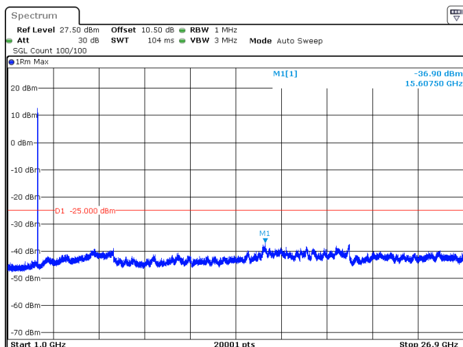
10MHz_30kHz_2685MHz_DFT-s-OFDM QPSK_RB24@0 -36.90 dBm
