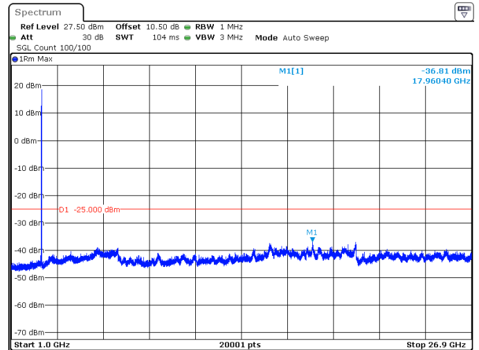
40MHz_30kHz_2670MHz_DFT-s-OFDM QPSK_RB1@105 -36.81 dBm
