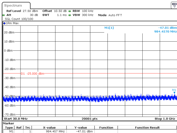
20MHz_30kHz_2679.99MHz_DFT-s-OFDM QPSK_RB1@50 -47.01 dBm
