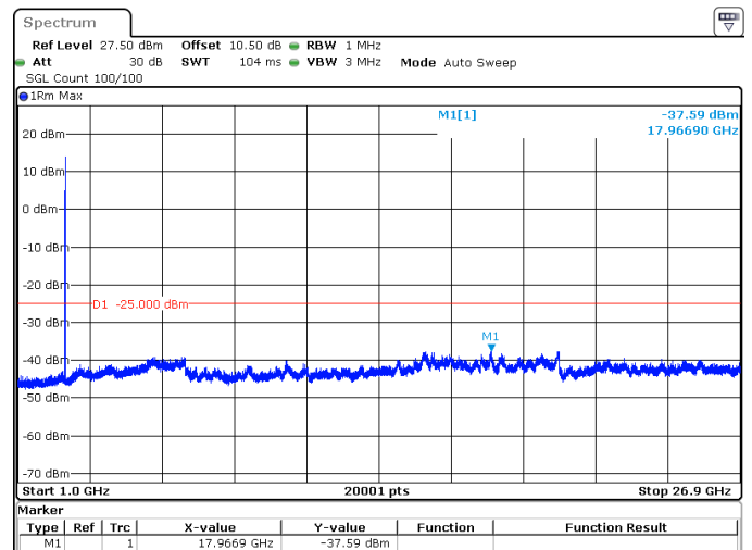
20MHz_30kHz_2679.99MHz_DFT-s-OFDM QPSK_RB1@50 -37.59 dBm
