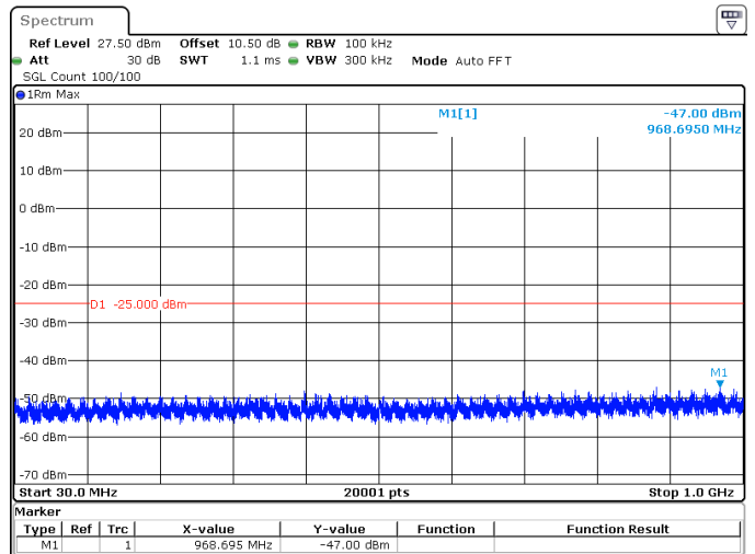
40MHz_15kHz_2593.005MHz_DFT-s-OFDM QPSK_RB1@0 -47.00 dBm
