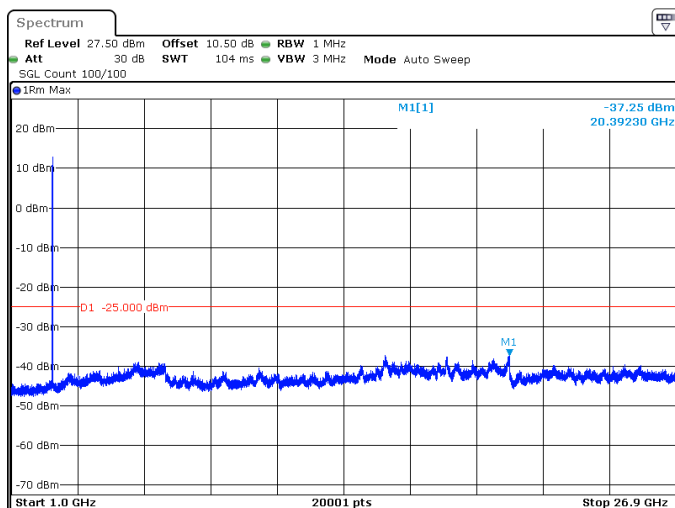
10MHz_30kHz_2592.99MHz_DFT-s-OFDM QPSK_RB24@0 -37.25 dBm
