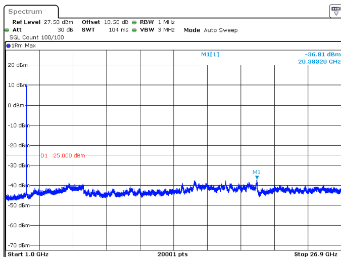
20MHz_30kHz_2592.99MHz_DFT-s-OFDM QPSK_RB50@0 -36.81 dBm
