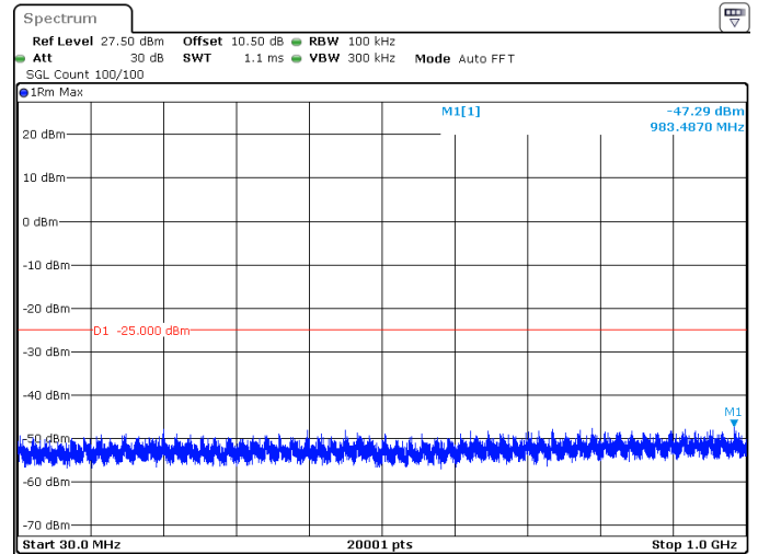
50MHz_30kHz_2521.02MHz_DFT-s-OFDM QPSK_RB1@0 -47.29 dBm
