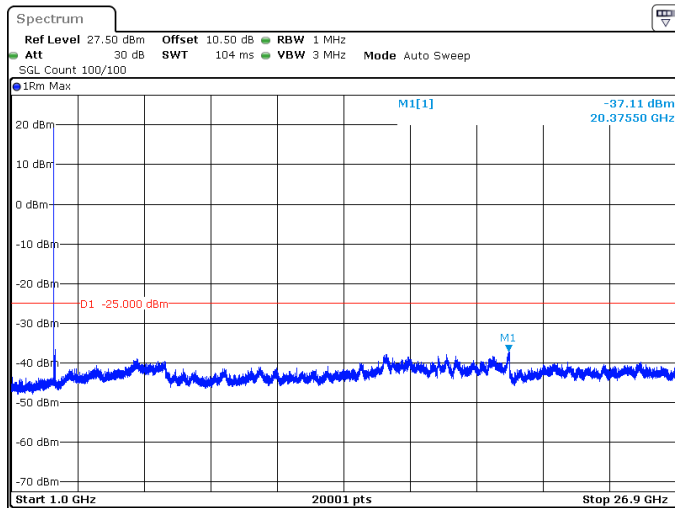
60MHz_30kHz_2659.98MHz_DFT-s-OFDM QPSK_RB1@0 -37.11 dBm
