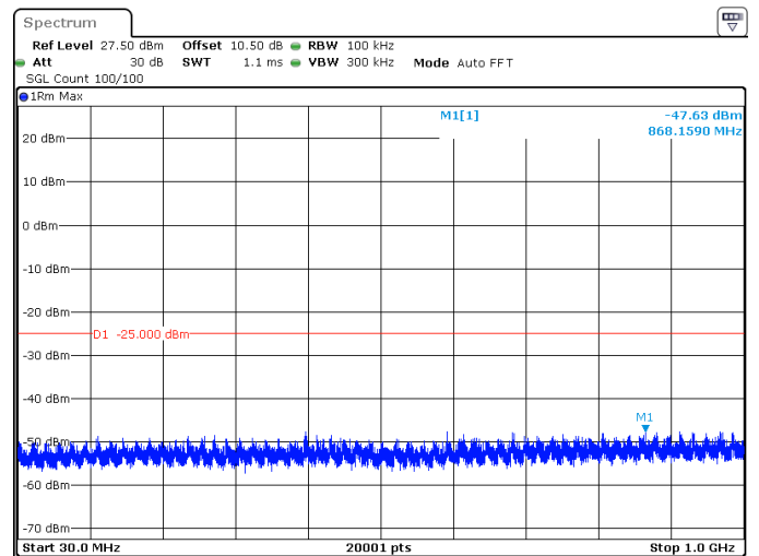
20MHz_30kHz_2592.99MHz_DFT-s-OFDM QPSK_RB1@50 -47.63 dBm
