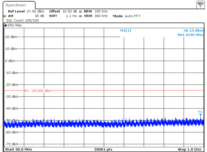
20MHz_15kHz_2593.005MHz_DFT-s-OFDM QPSK_RB1@0 -46.13 dBm
