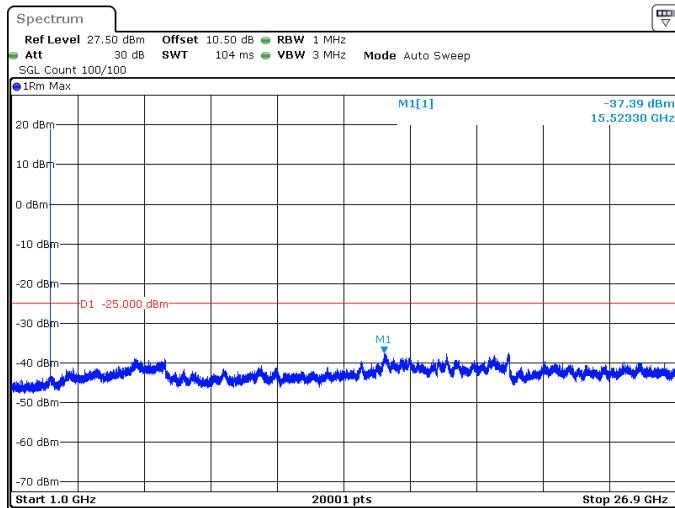
20MHz_15kHz_2506.005MHz_DFT-s-OFDM QPSK_RB1@0 -37.39 dBm
