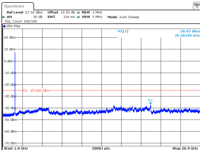
40MHz_15kHz_2593.005MHz_DFT-s-OFDM QPSK_RB216@0 -36.82 dBm
