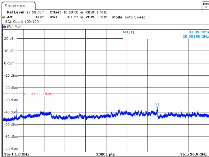
40MHz_30kHz_2670MHz_DFT-s-OFDM QPSK_RB1@0 -37.09 dBm
