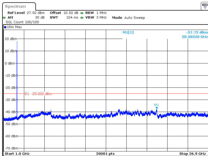
10MHz_30kHz_2685MHz_DFT-s-OFDM QPSK_RB1@23 -37.72 dBm
