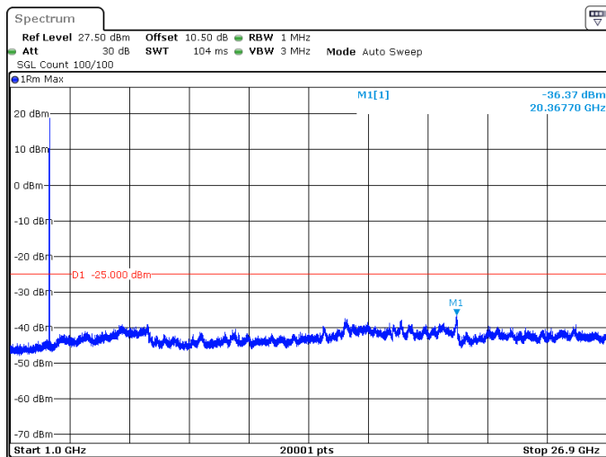
15MHz_30kHz_2682.48MHz_DFT-s-OFDM QPSK_RB1@37 -36.37 dBm
