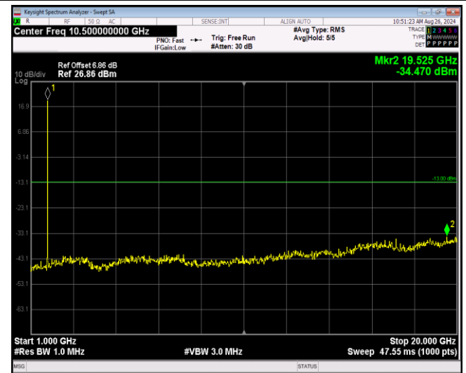
Band4-1.4MHz-16QAM-19957-1RB#0-Range2:1000~2 0000MHz
