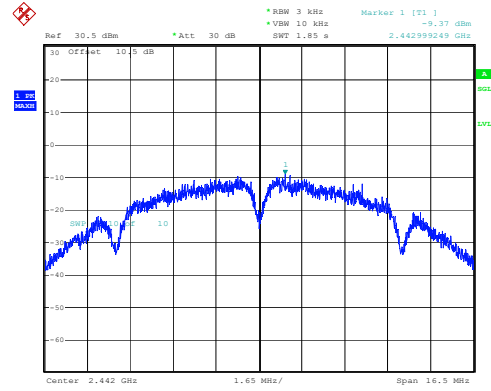
802.11b_2442MHz
