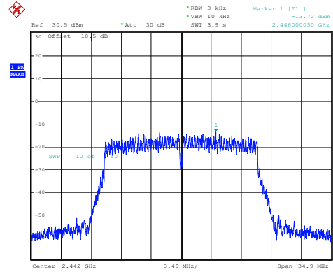
802.11n20_2442MHz
