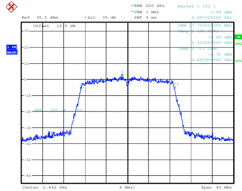
802.11n20_2442MHz
