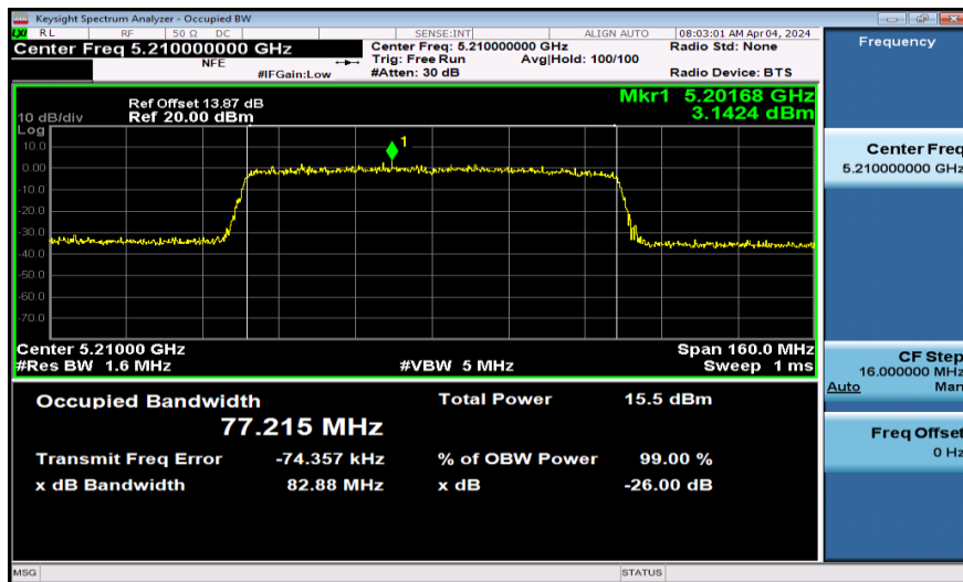
11AX80SISO-Ant1-5210
