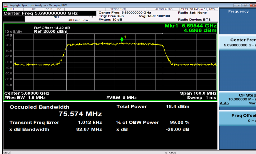
11AC80SISO-Ant1-5690
