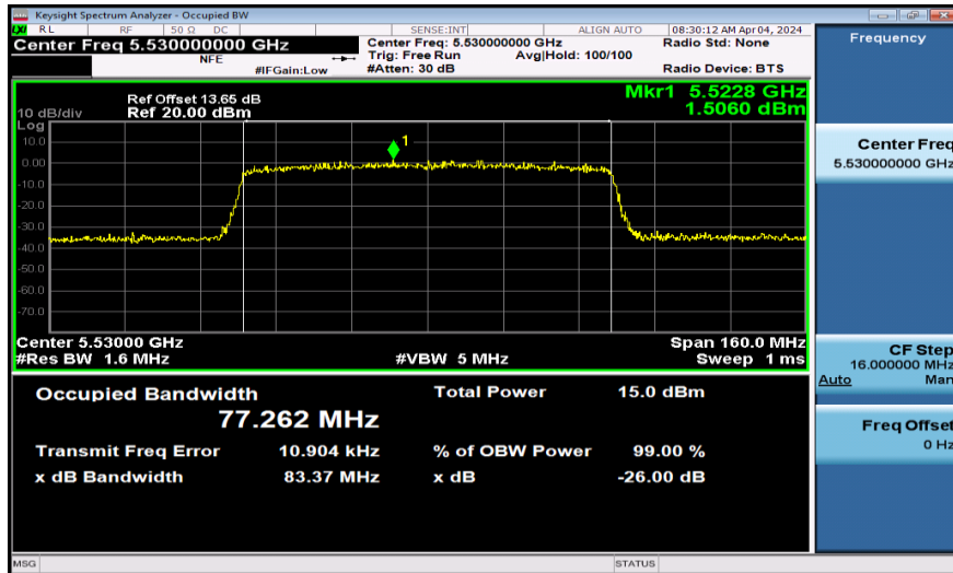
11AX80SISO-Ant1-5530
