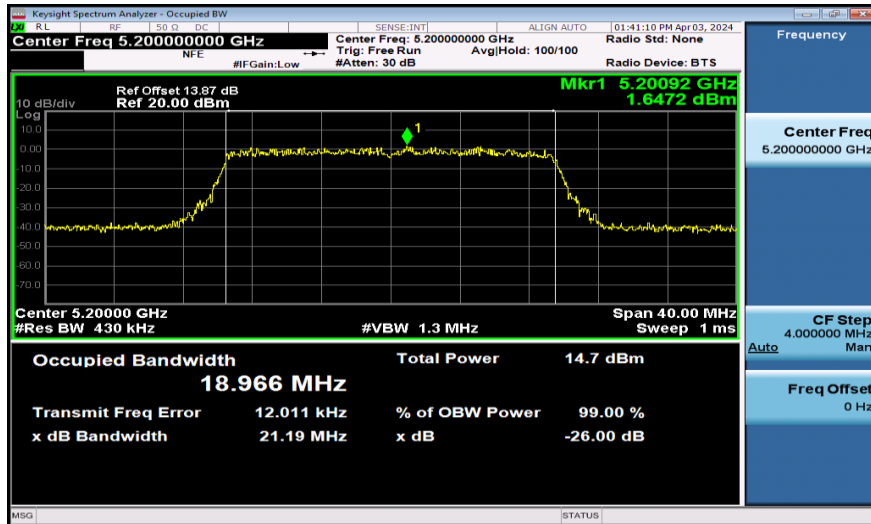
11AX20SISO-Ant1-5200
