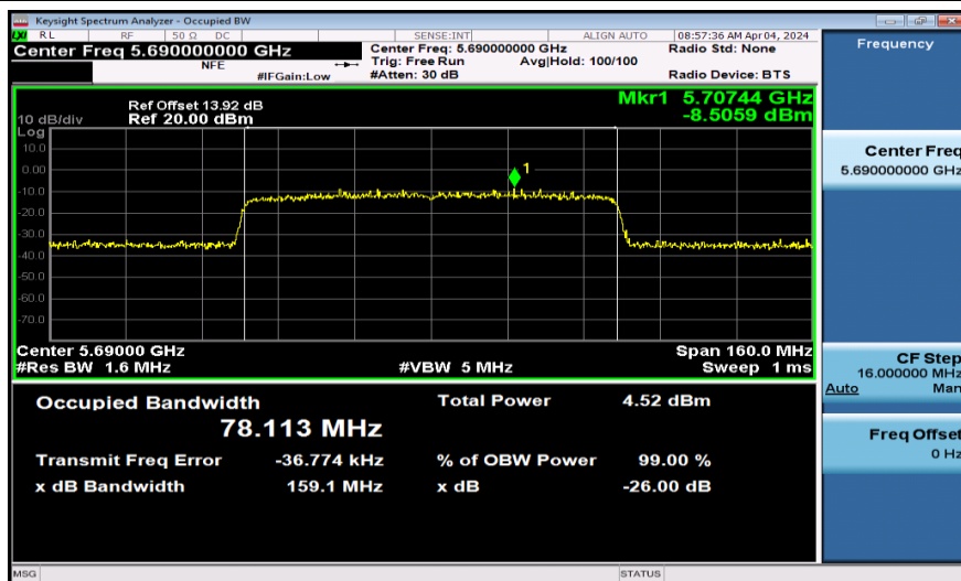
11AX80SISO-Ant1-5690
