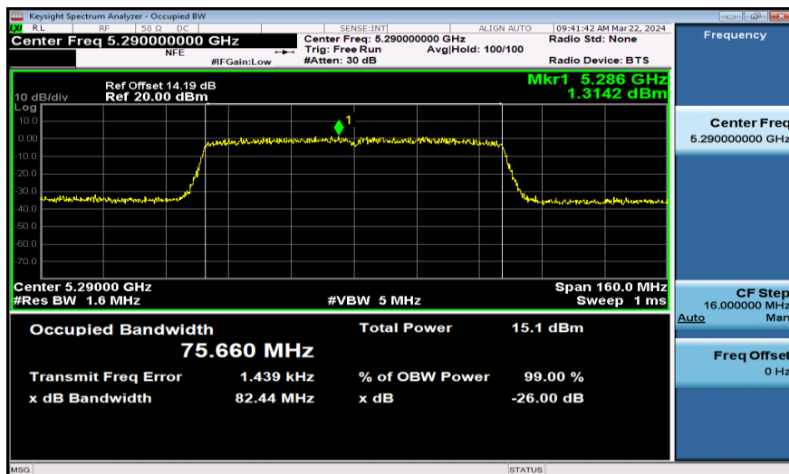
11AC80SISO-Ant1-5290
