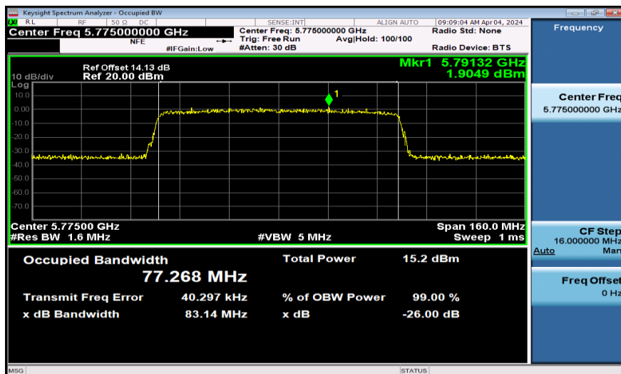
11AX80SISO-Ant1-5775
