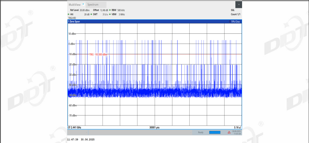
3DH3_Ant1_Hop
