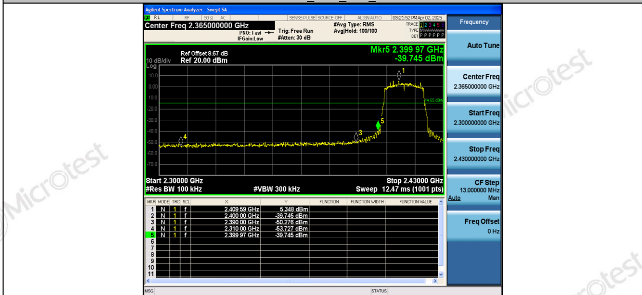
11N20SISO_Ant2_Low_2412
