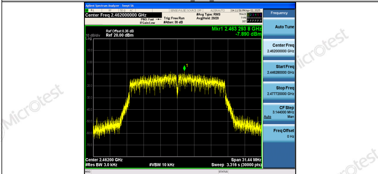
11N20MIMO_Ant2_2462
