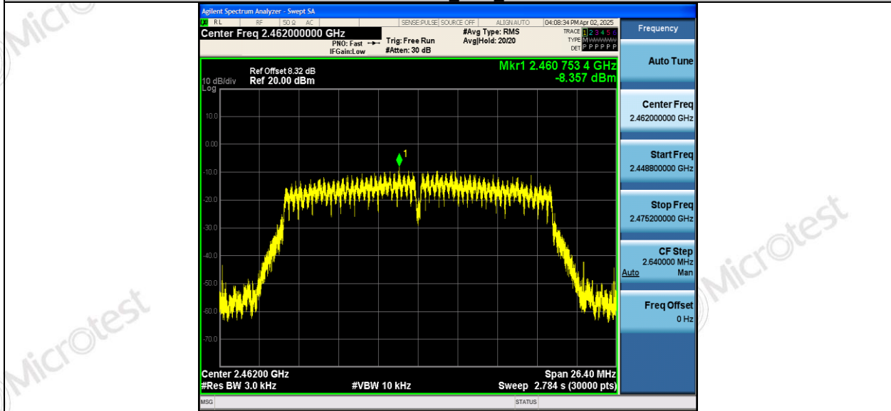
11N20MIMO_Ant2_2462
