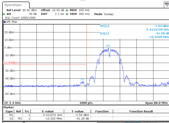
802.11b_2412MHz
