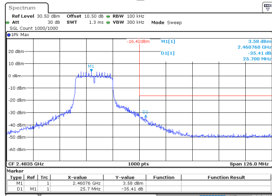
802.11n20_2462MHz
