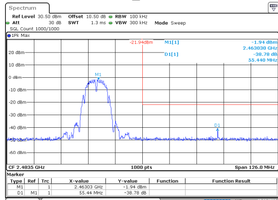
802.11b_2462MHz
