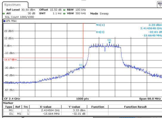
802.11n20_2412MHz
