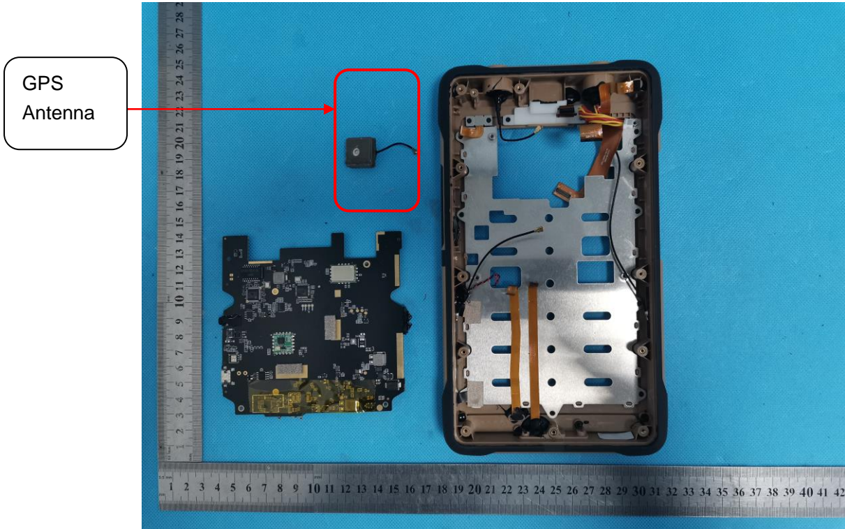
GPS ANTENNA
