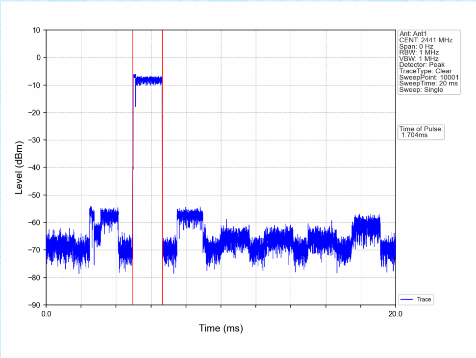
Pi/4DQPSK_2DH3_HOPP_Ant1_NTNV
