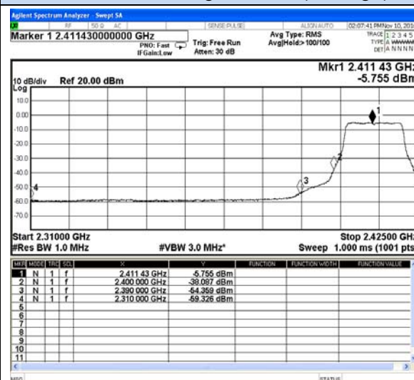
802.11g-Low channel(Average)
