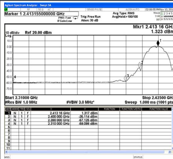
802.11b-Low channel(Average)
