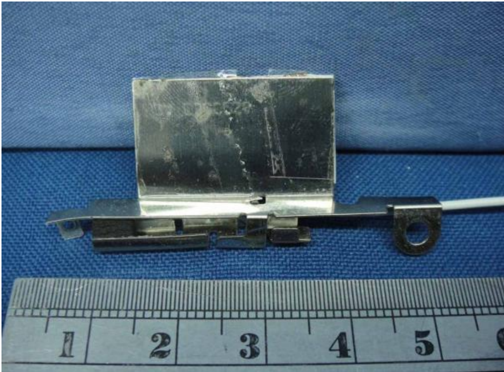
(5) EUT Photo
