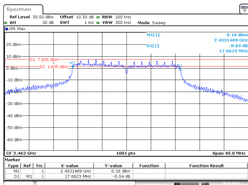
n20_2462MHz_Chain 0
