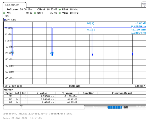
b_2437MHz_Chain 0
