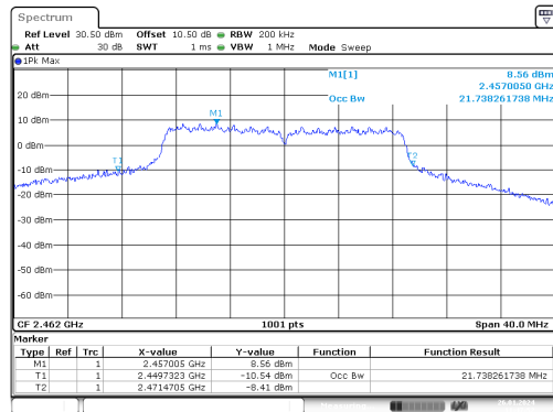
n20_2462MHz_Chain 0
