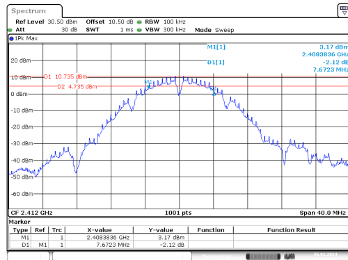
b_2412MHz_Chain 0
