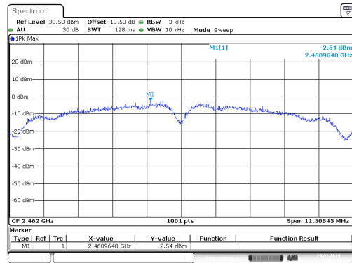
b_2462MHz_Chain 0
