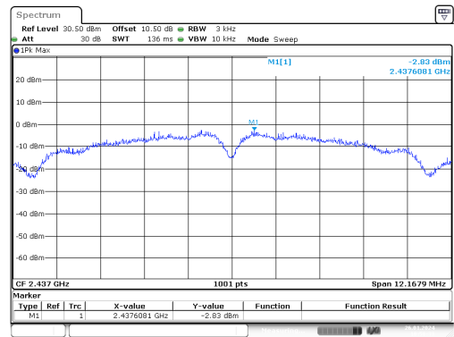
b_2437MHz_Chain 0
