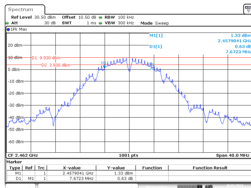
b_2462MHz_Chain 0
