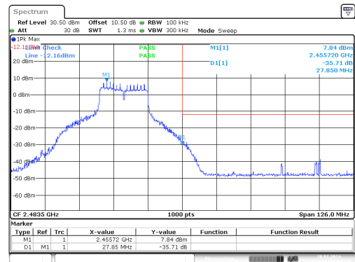
n20_2462MHz_Chain 0
