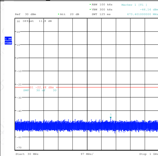
BLE_2M-Ant1-2440-30~1000-PASS
