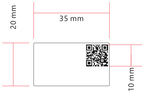
尺寸图 A-图
