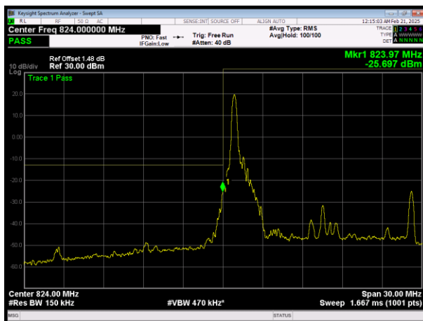
LLTE Band26 (824-849) QAM16 BW=15MHz Channel=26865 RB Size=1 Position=#0
