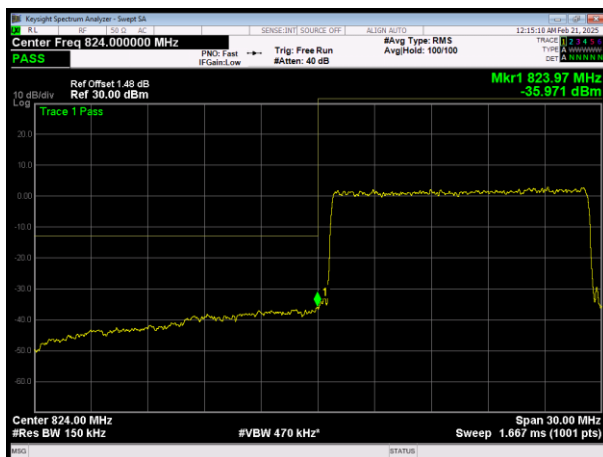
LLTE Band26 (824-849) QAM16 BW=15MHz Channel=26865 RB Size=75 Position=#0
