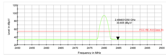
BLE Channel 39 Average
