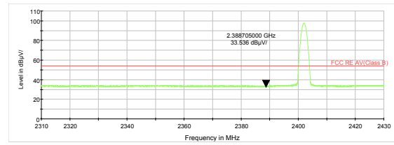
BLE Channel 0 Average
