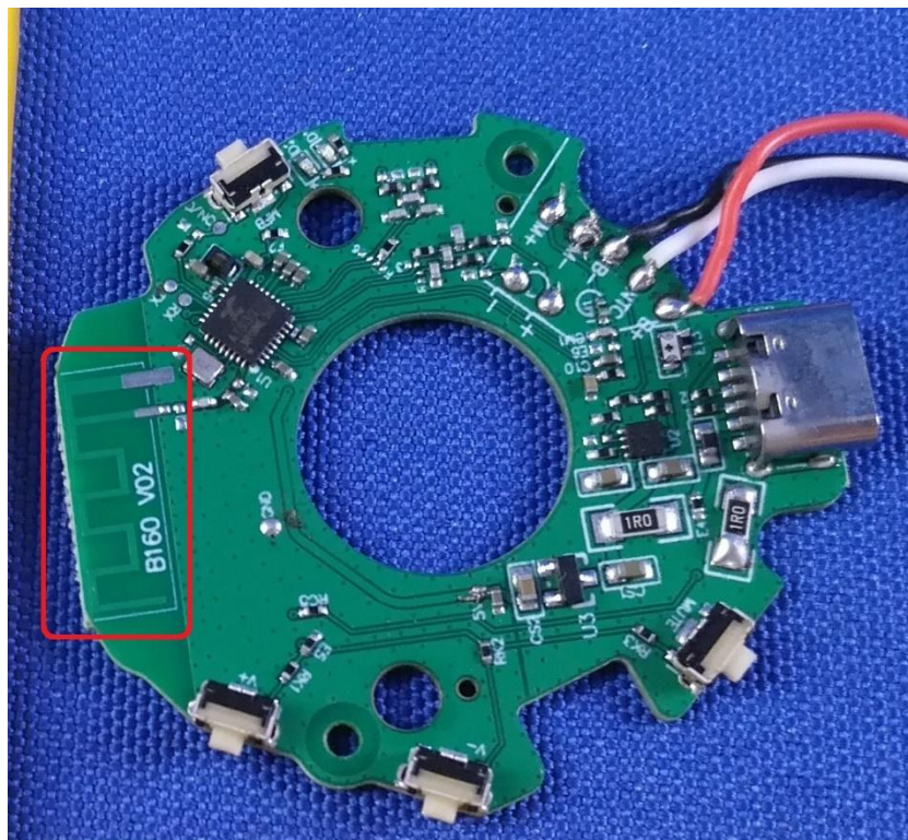
Antenna
