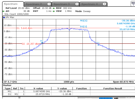
n20_5700MHz_Chain 0
