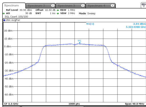
n20_5500MHz_Chain 0
