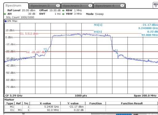
ac80_5290MHz_Chain 0
