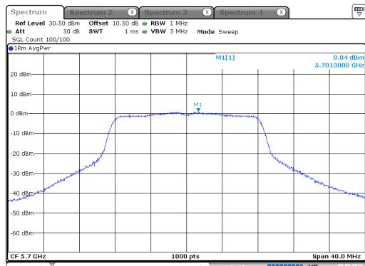
a_5700MHz_Chain 0
