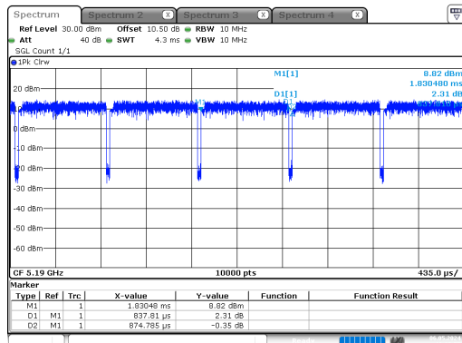
n40_5190MHz_Chain 0
