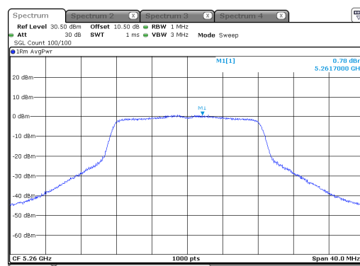
a_5260MHz_Chain 0
