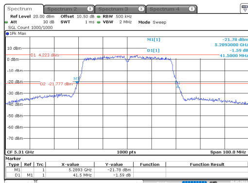
n40_5310MHz_Chain 0
