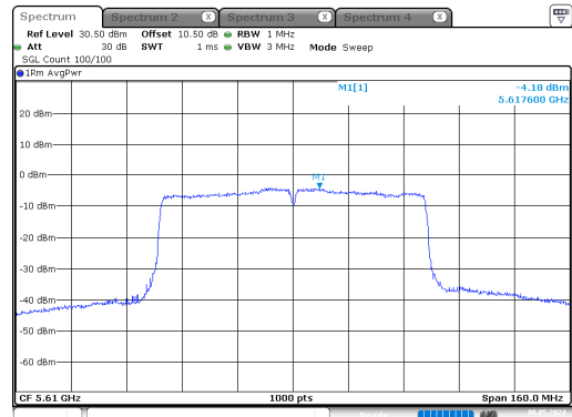
ac80_5610MHz_Chain 0
