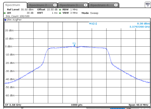
a_5580MHz_Chain 0
