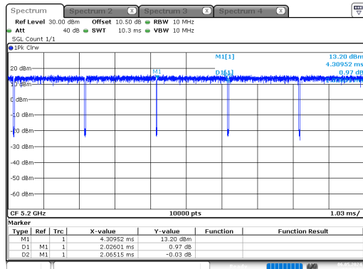
a_5200MHz_Chain 0
