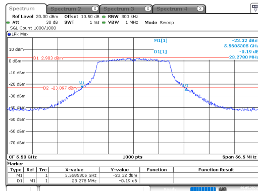
a_5580MHz_Chain 0
