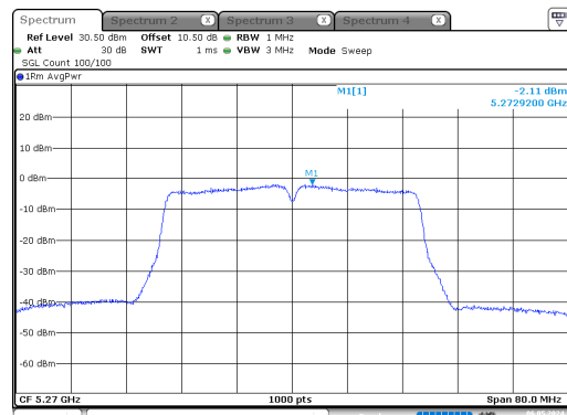
n40_5270MHz_Chain 0
