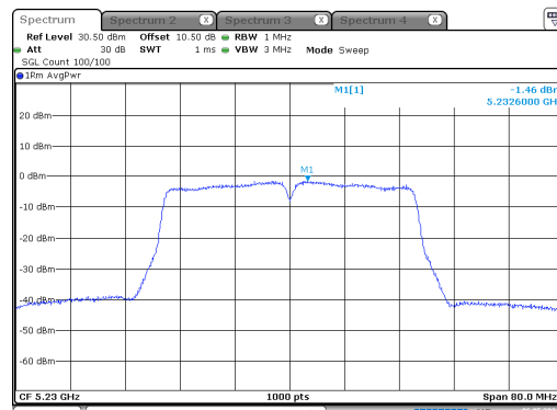
n40_5230MHz_Chain 0
