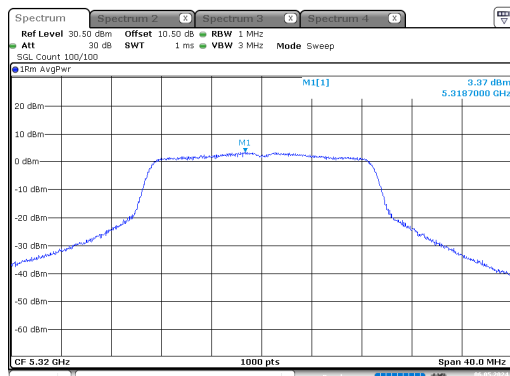
n20_5320MHz_Chain 0
