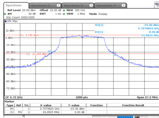
a_5720MHz_Chain 0
