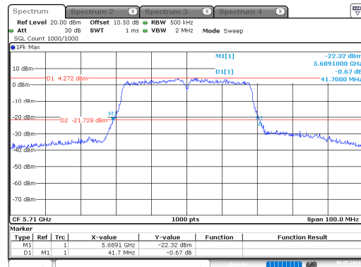
n40_5710MHz_Chain 0
