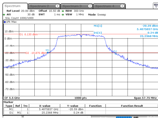
n20_5500MHz_Chain 0
