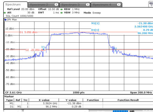
ac80_5610MHz_Chain 0
