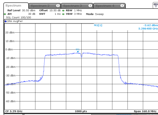
ac80_5290MHz_Chain 0
