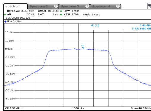
a_5320MHz_Chain 0
