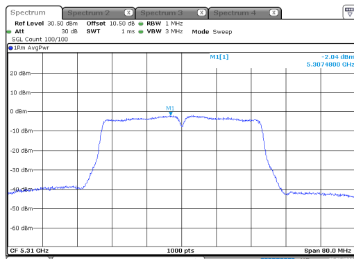
n40_5310MHz_Chain 0
