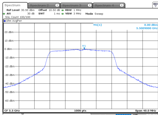
a_5500MHz_Chain 0
