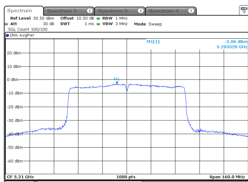
ac80_5210MHz_Chain 0
