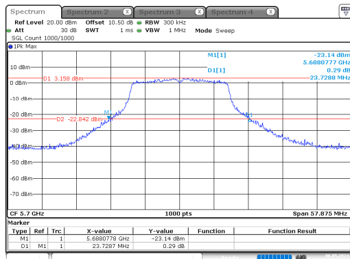
a_5700MHz_Chain 0
