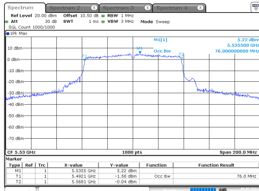
ac80_5530MHz_Chain 0
