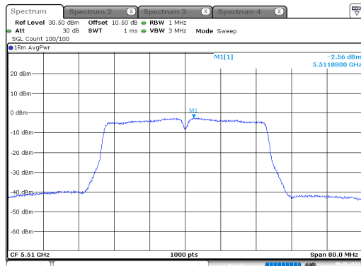
n40_5510MHz_Chain 0
