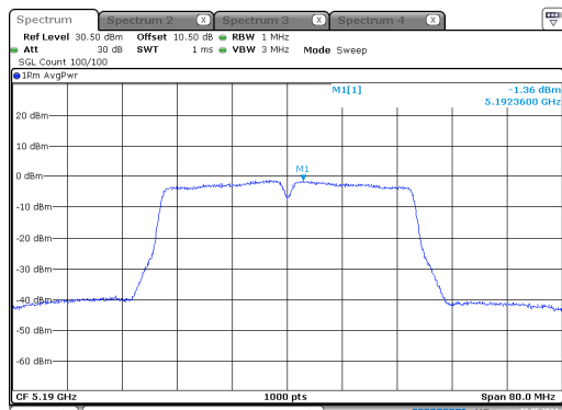
n40_5190MHz_Chain 0
