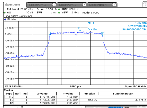
n40_5755MHz_Chain 0
