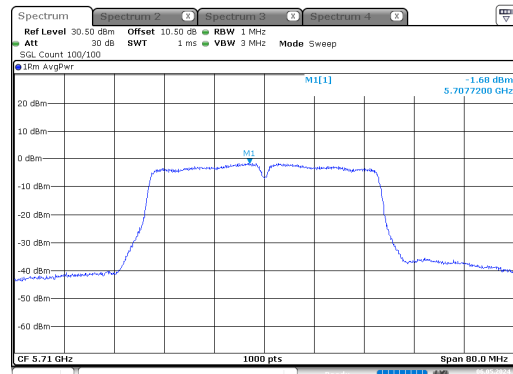
n40_5710MHz_Chain 0
