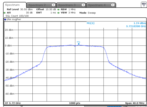
a_5720MHz_Chain 0
