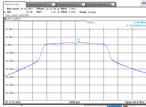
n20_5720MHz_Chain 0
