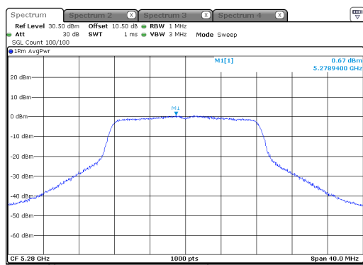
a_5280MHz_Chain 0
