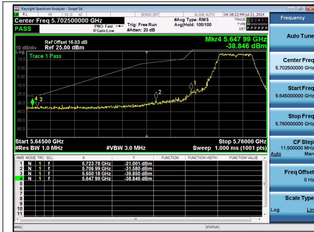
11A-Ant0-5745-PASS
