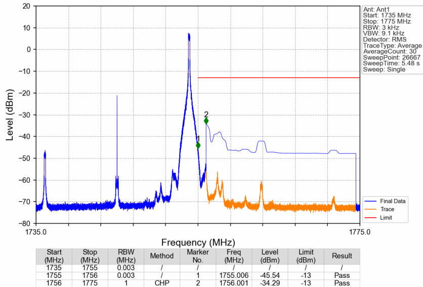
Band4_20MHz_QPSK_HCH_1745MHz_RB_1_99_NTNV
