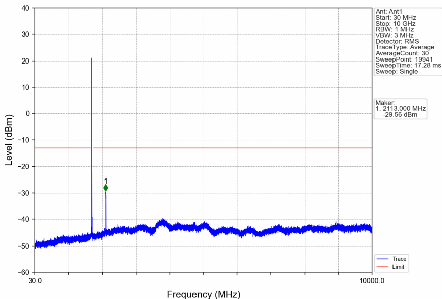
Band4_20MHz_16QAM_LCH_1720MHz_RB_1_0_NTNV
