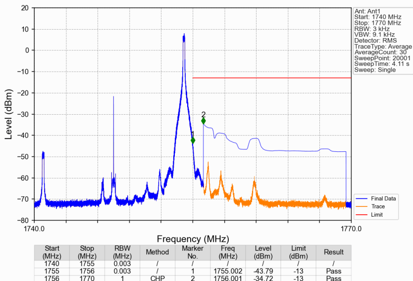
Band4_15MHz_QPSK_HCH_1747.5MHz_RB_1_74_NTNV
