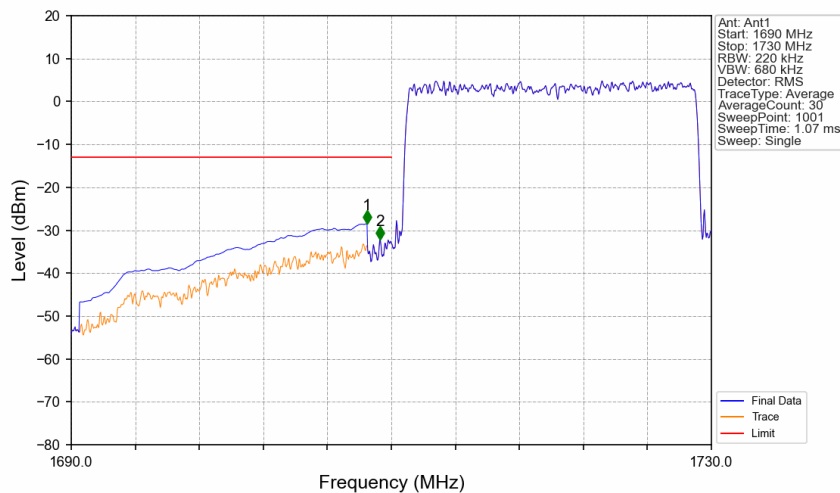
Band4_20MHz_QPSK_LCH_1720MHz_RB_100_0_NTNV
