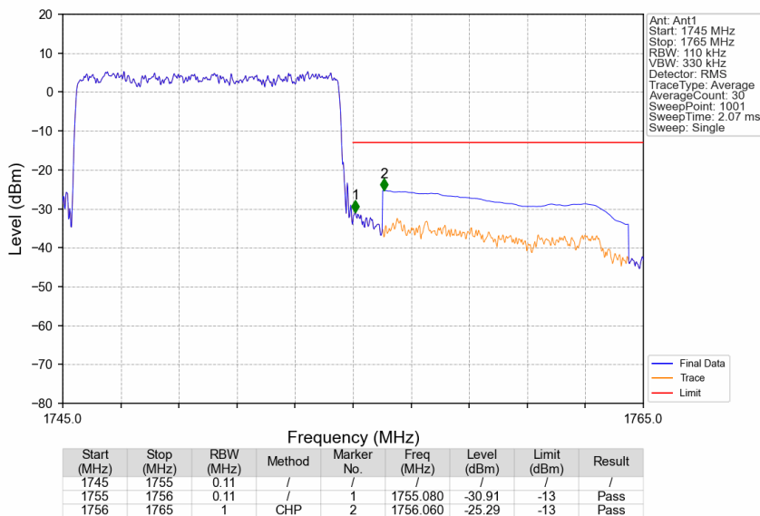
Band4_10MHz_QPSK_HCH_1750MHz_RB_50_0_NTNV
