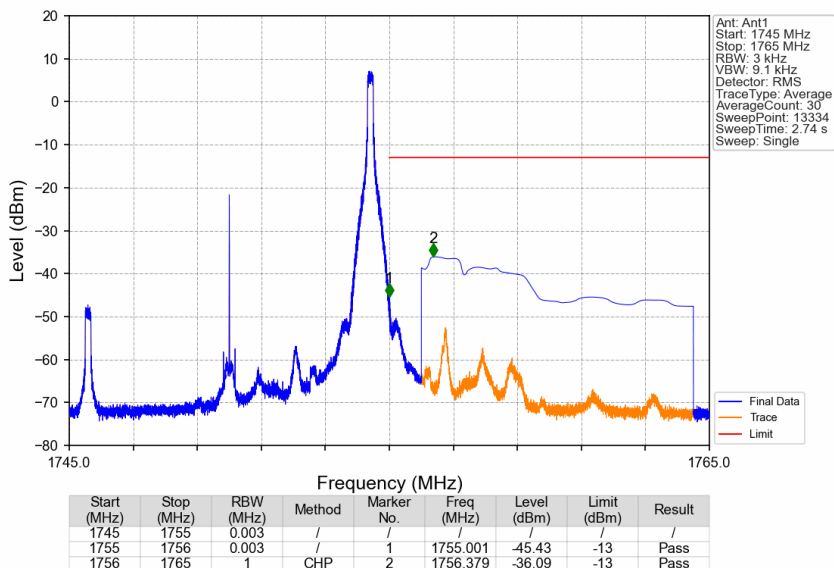
Band4_10MHz_QPSK_HCH_1750MHz_RB_1_49_NTNV
