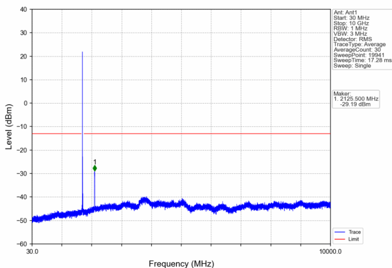
Band4_20MHz_QPSK_LCH_1720MHz_RB_1_0_NTNV
