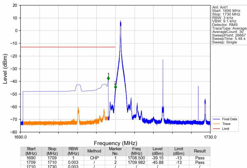
Band4_20MHz_QPSK_LCH_1720MHz_RB_1_0_NTNV
