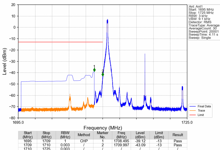
Band4_15MHz_QPSK_LCH_1717.5MHz_RB_1_0_NTNV
