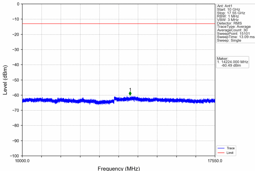
Band4_20MHz_16QAM_LCH_1720MHz_RB_100_0_NTNV
