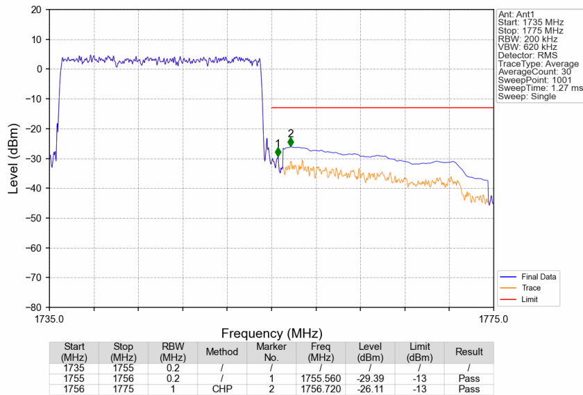
Band4_20MHz_QPSK_HCH_1745MHz_RB_100_0_NTNV
